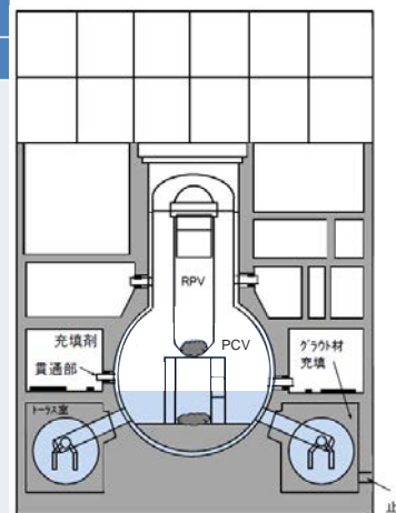
原子炉格納容器下部水張りイメージ図
