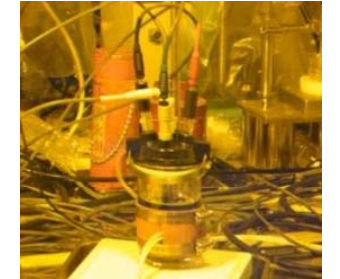
照射済被覆管の電気化学試験
