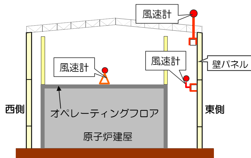
風速測定イメージ
