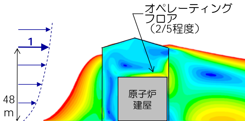
屋根パネル2枚外した状態（東風）
