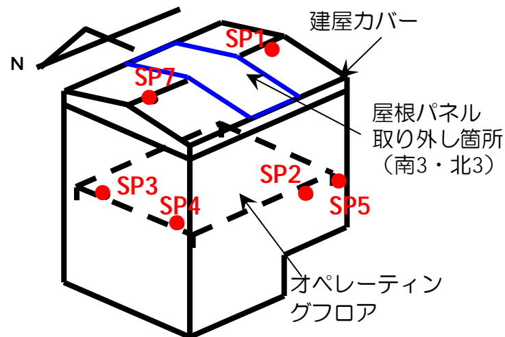
ダストモニタのサンプリング箇所
