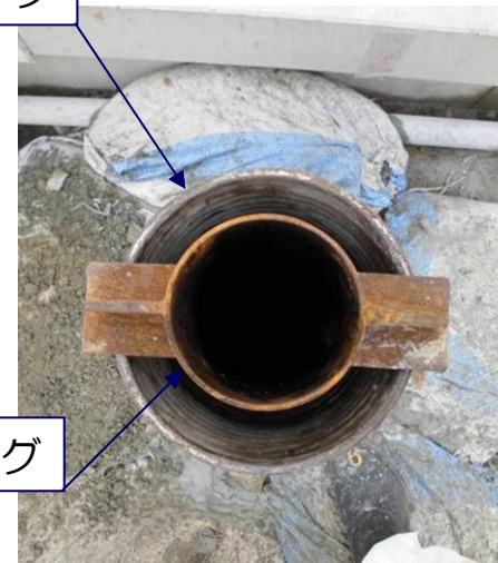
二重管設置
