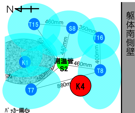
O.P.+0.4m付近
