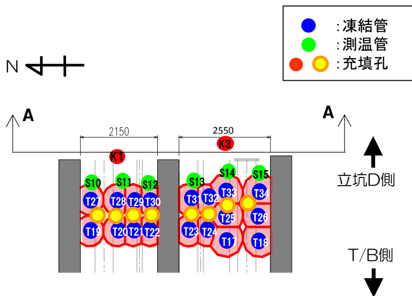
平面図
