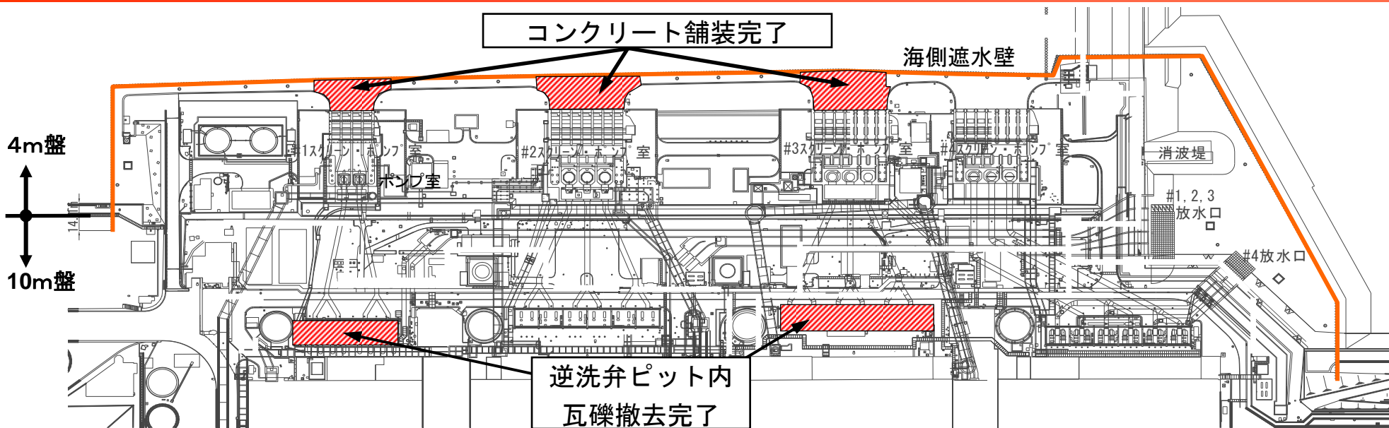
逆洗弁ピット(3号)内瓦礫撤去完了
