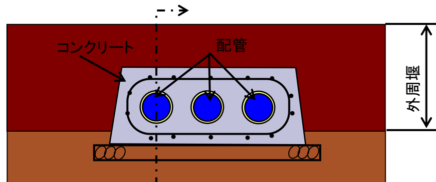
断面図
