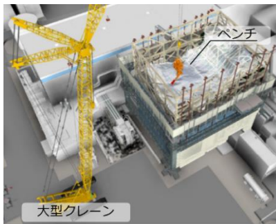
<1-10. クレーン吊り遠隔操作イメージ>
