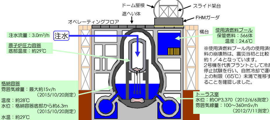
<1-28. プラント関連パラメータ>
