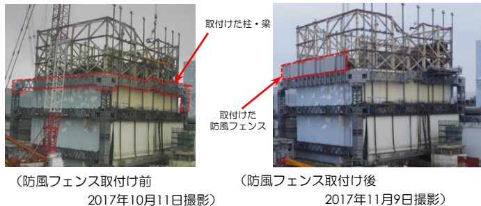
<1-1. 防風フェンス設置状況>
