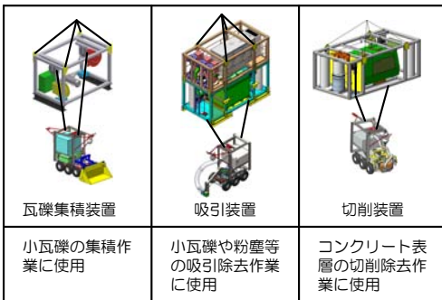
自走式除染装置
