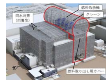
燃料取り出し用カバーイメージ
