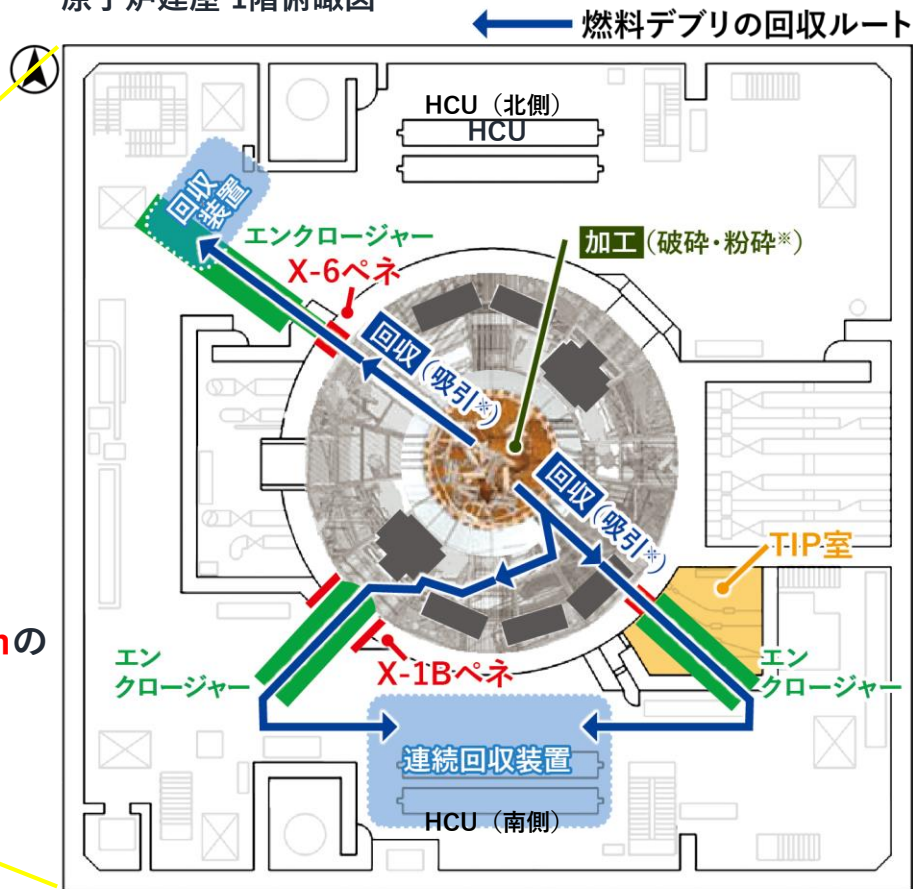
原子炉建屋 1階俯瞰図
