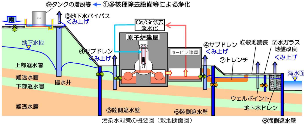
汚染水対策の概要図（敷地断面図）
