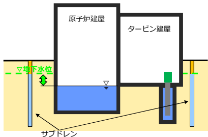
<2-3. 1号建屋滞留水と地下水位の管理 (イメージ)>
