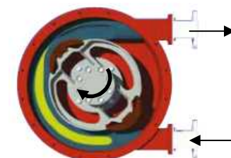
ブースターポンプ作動イメージ
