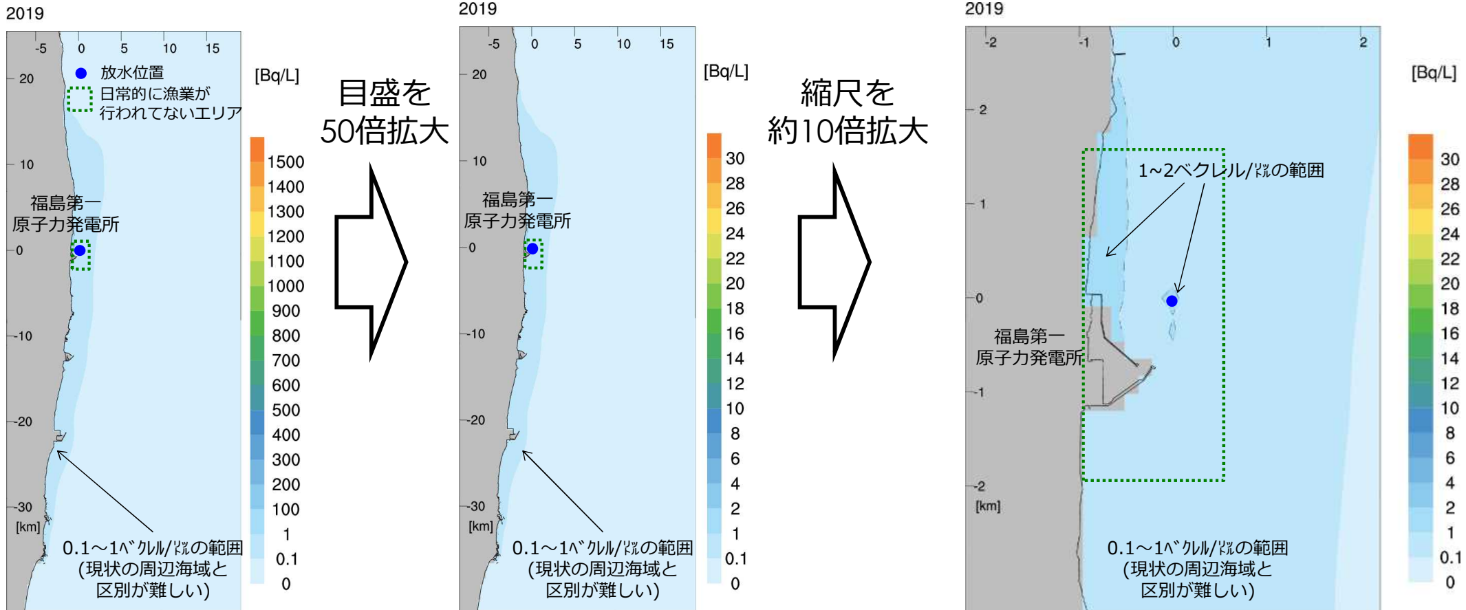
福島県沖拡大図 (最大目盛30ベクレル/ℓにて作図)
