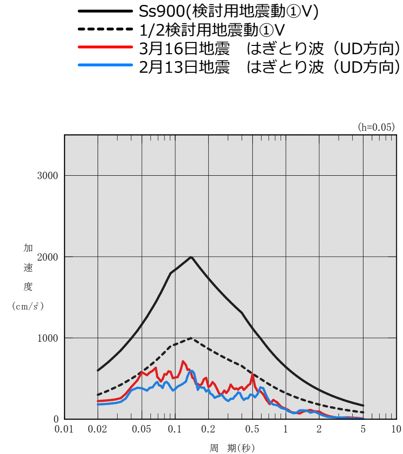
はぎとり波と検討用地震動の比較 (鉛直方向)
