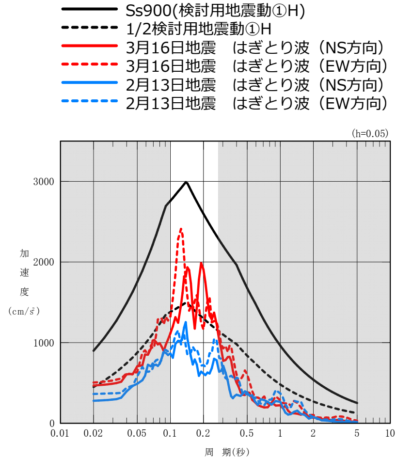
はぎとり波と検討用地震動の比較 (水平方向)
