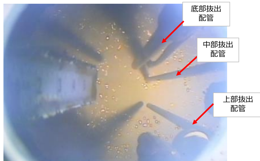
SEDS付属のカメラによるスラリー移送直後の 移送元HIC内画像
