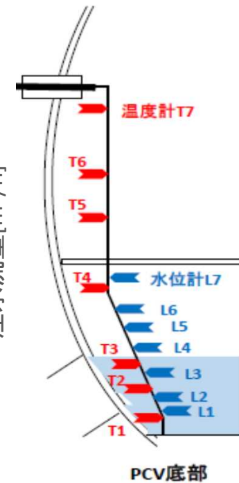
PCV底部 温度計の設置概要
