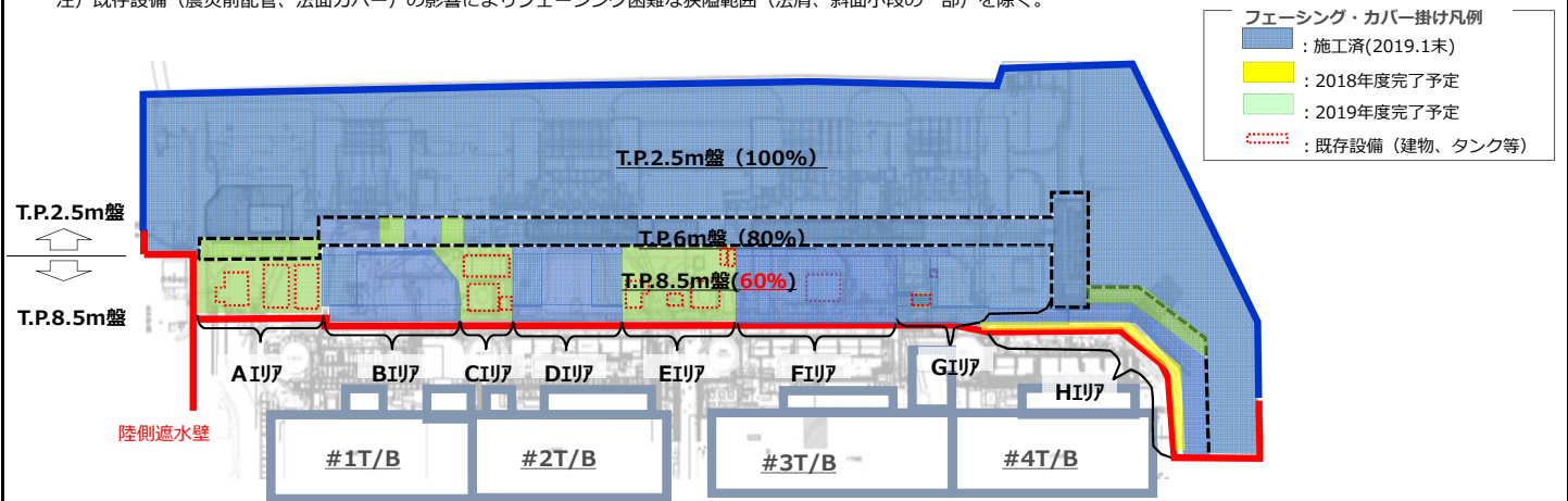
フェーシングエリア配置図
