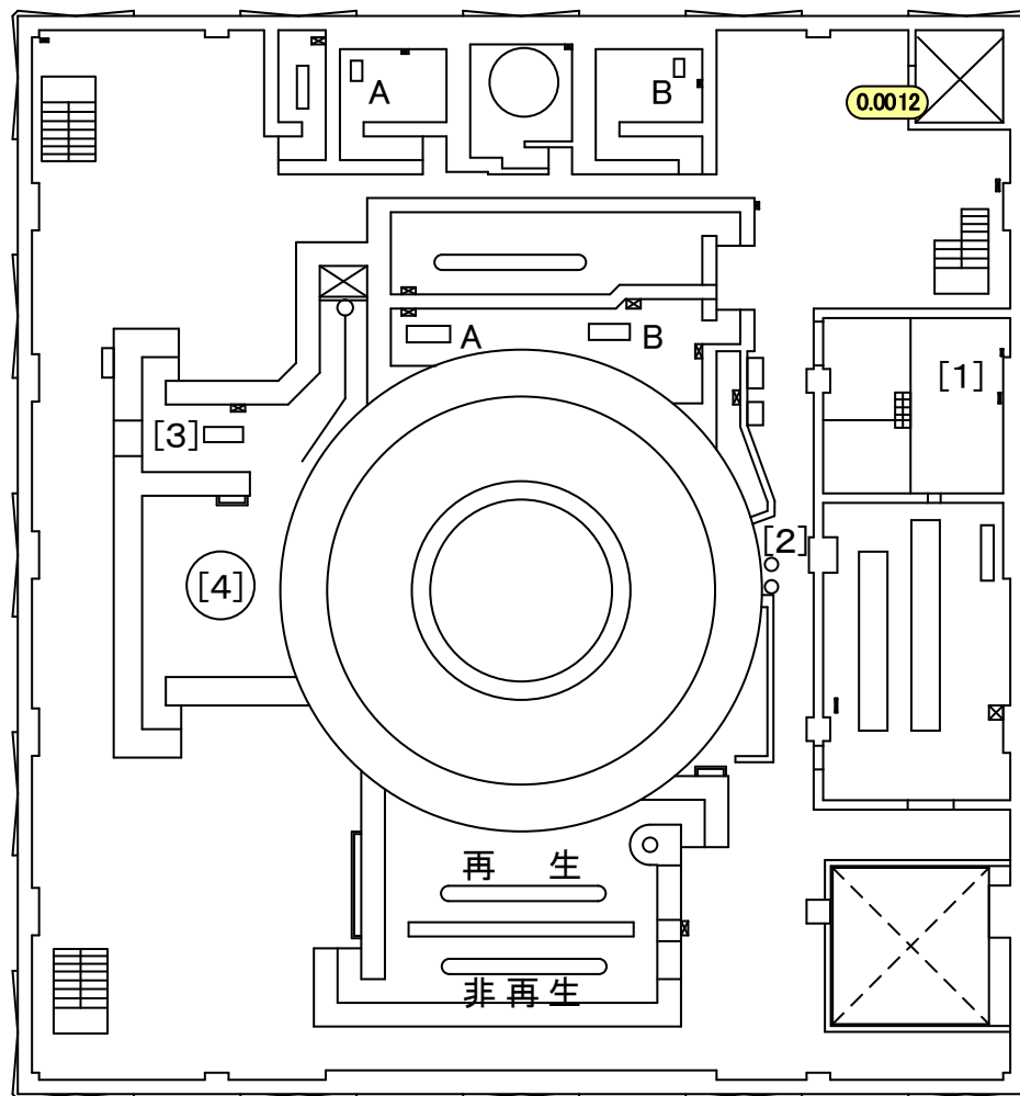
CUW逆洗水移送ポンプ
