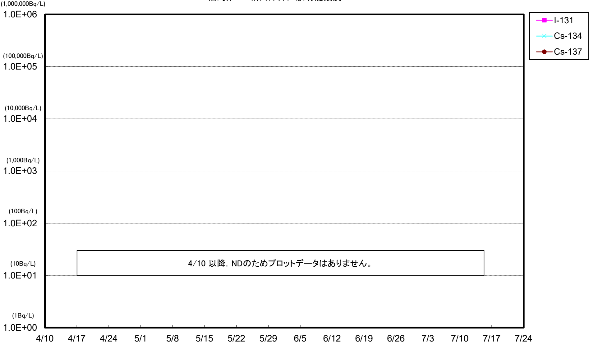
福島第一 構内深井戸放射能濃度
