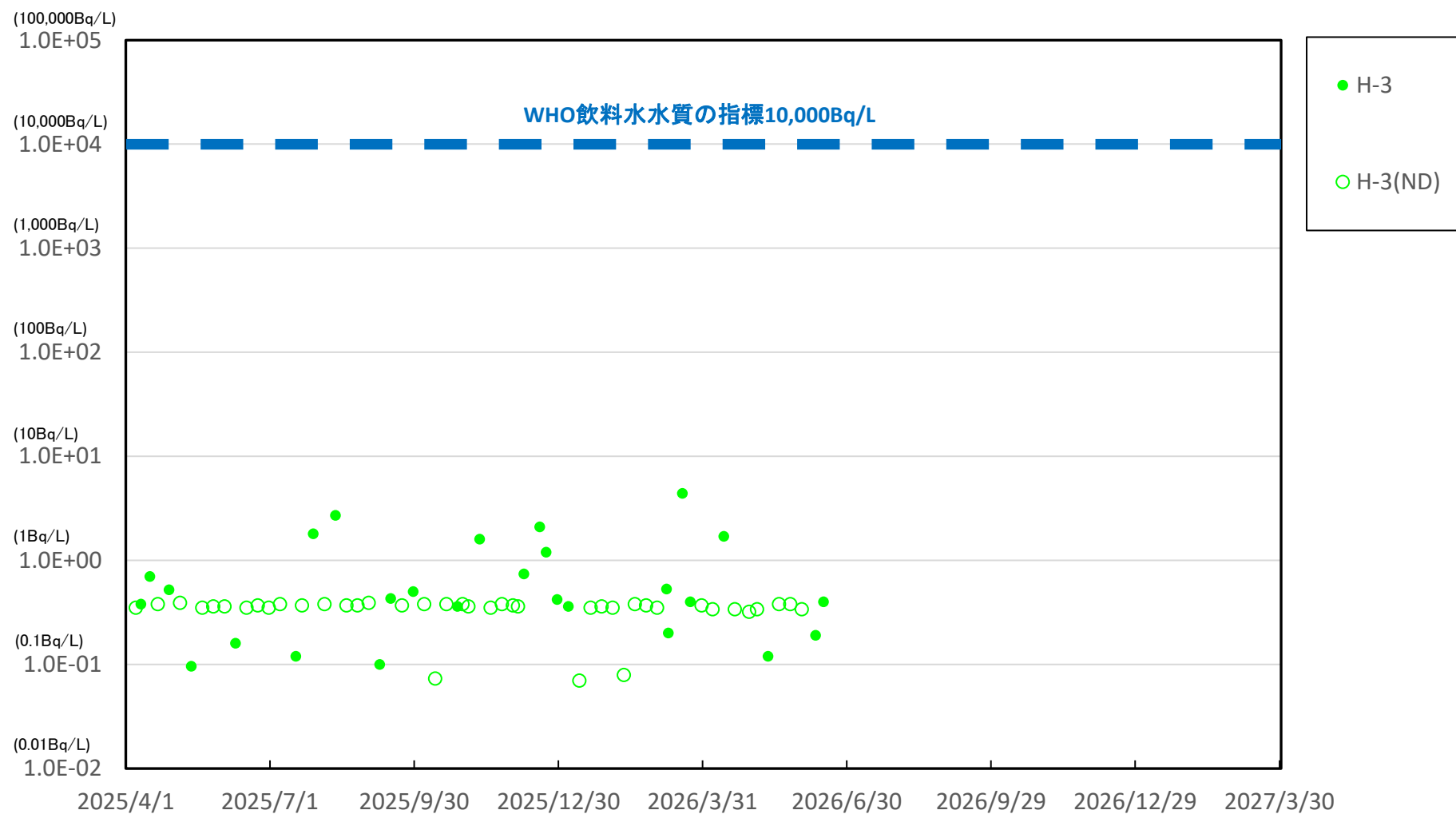
1F敷地北側沖合1.5km(T-A1) 海水放射能濃度
