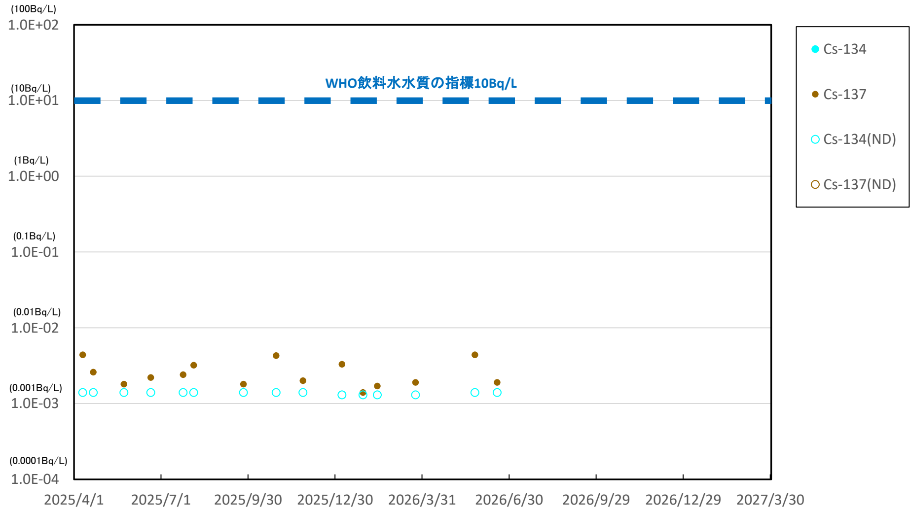
いわき市北部沖合3km(T-12) 表層 海水放射能濃度
