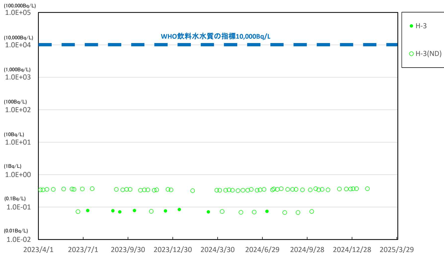
福島第一 敷地沖合15km(T-5) 表層 海水放射能濃度
