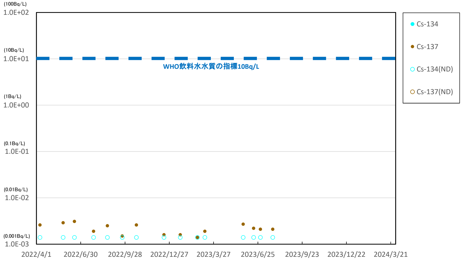
夏井川沖合1km(T-17-1) 底層 海水放射能濃度(Bq/L)
