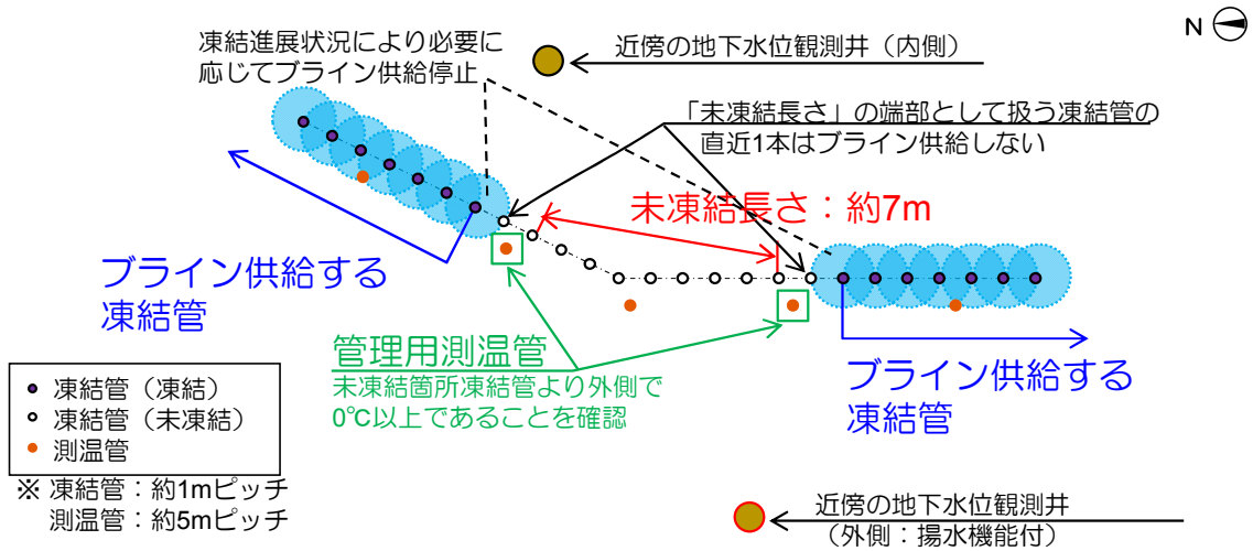
図-15 未凍結長さの管理図(例：西側③)
