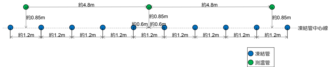
図－14 測温管の基本配置（海側の例）
