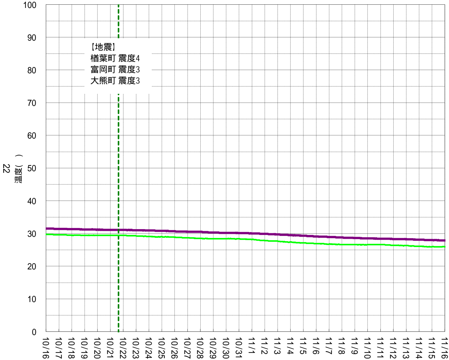
2号機 実施計画関連温度計(RPV)
