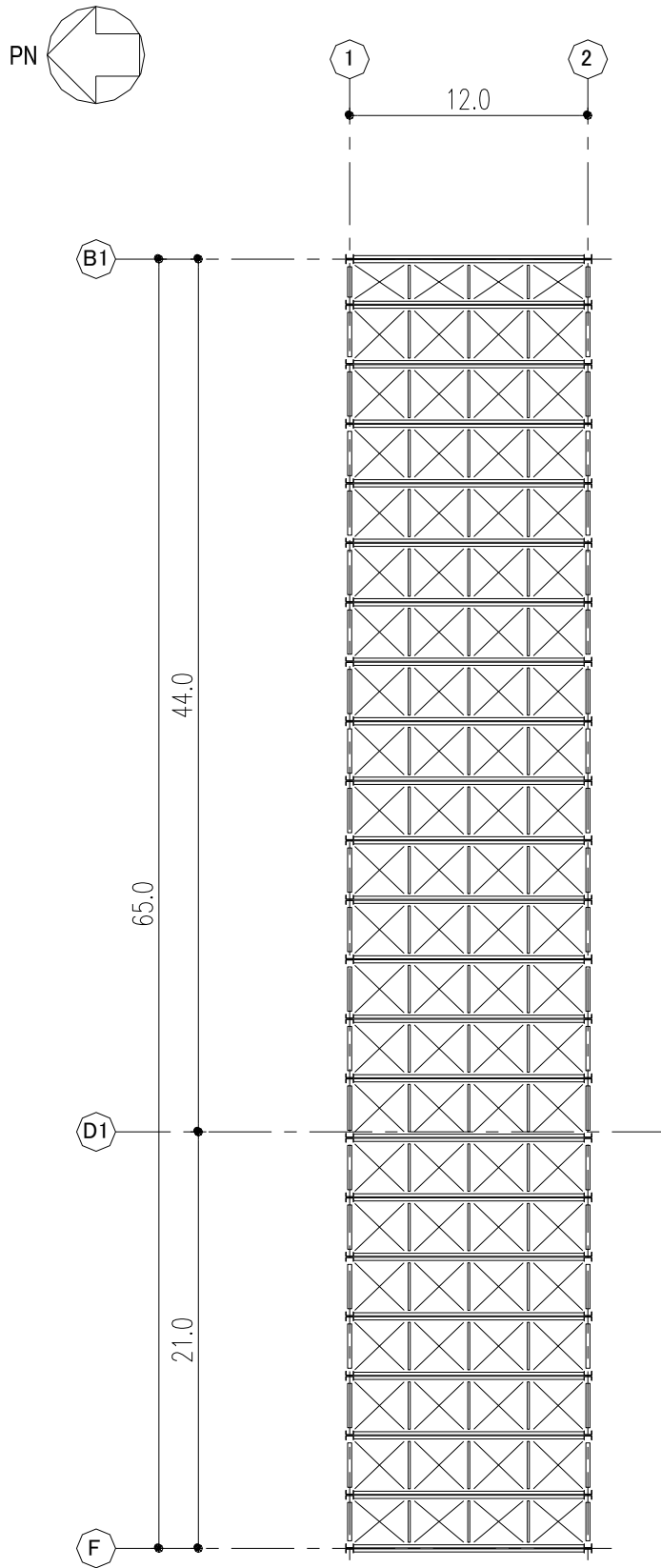
图-14 設備棟 屋根平面図 (O.P. 41.0) (単位:m)
