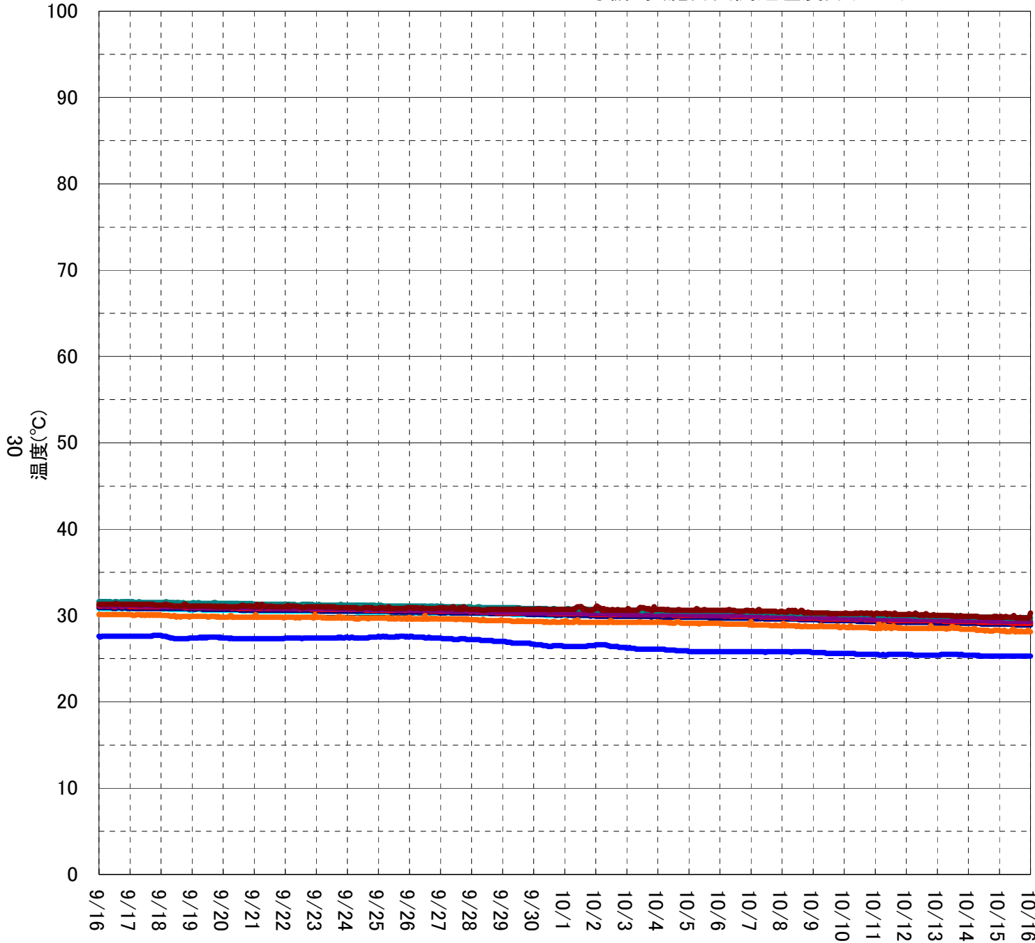
3号機 実施計画関連温度計(PCV)
