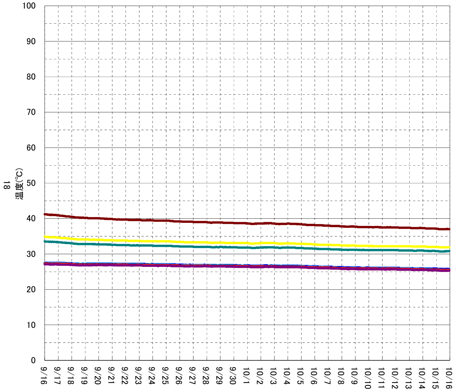
1号機 実施計画関連温度計(PCV)
