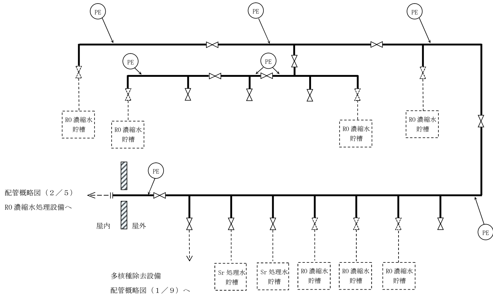
図-7 配管概略図 (1 / 5)
