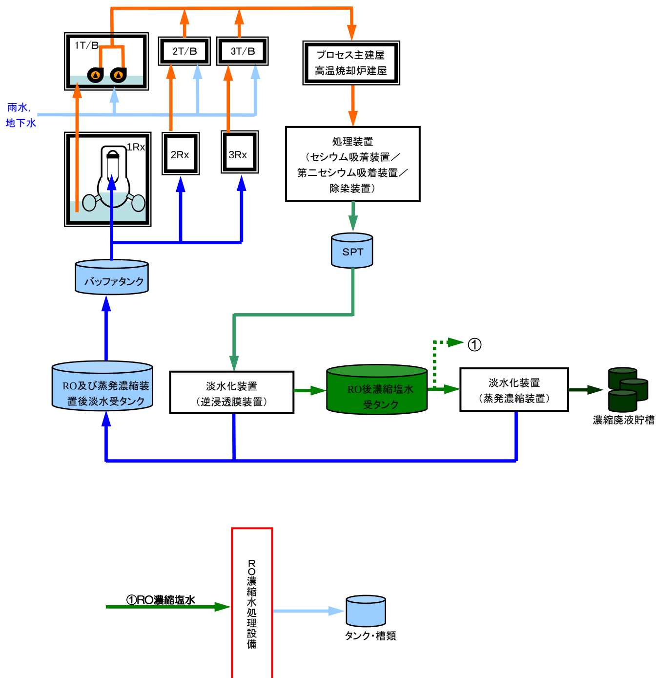
図－ 1 汚染水処理設備並びに RO 濃縮水処理設備等の全体概要図
