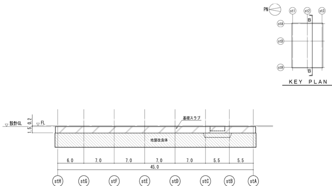
図－3 B-B 断面図 (EW 方向) (単位 : m)
