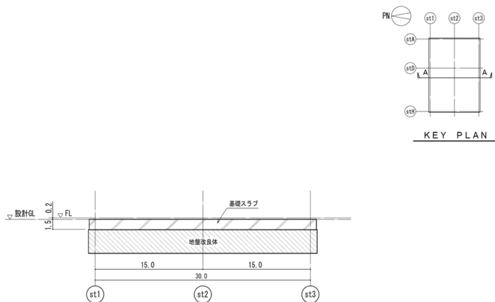
図－2 A-A 断面図 (NS 方向) (単位 : m)
