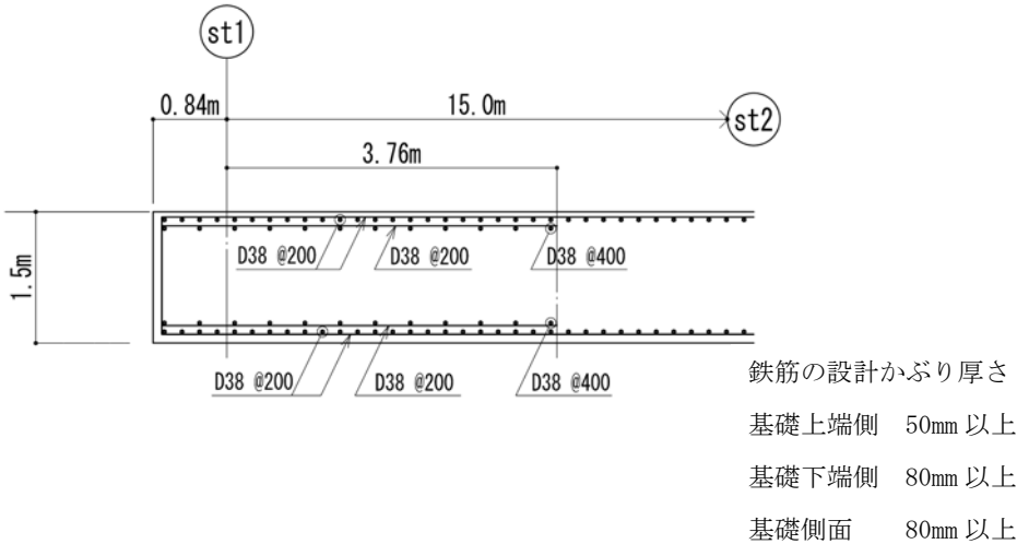
図－4 基礎スラブの配筋図 (stA通り)
