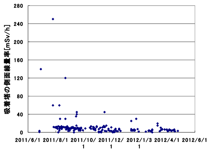
図 2 一時保管施設に保管したセシウム吸着装置吸着塔の発生時期と側面線量率分布
