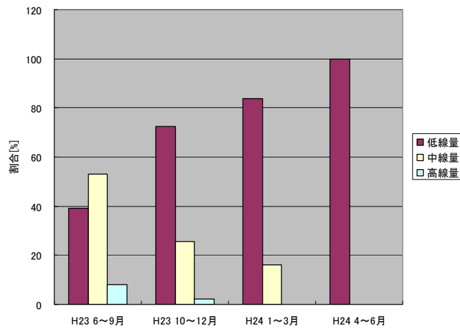
図 1 一時保管施設に保管したセシウム吸着装置吸着塔の発生時期による割合の変化
