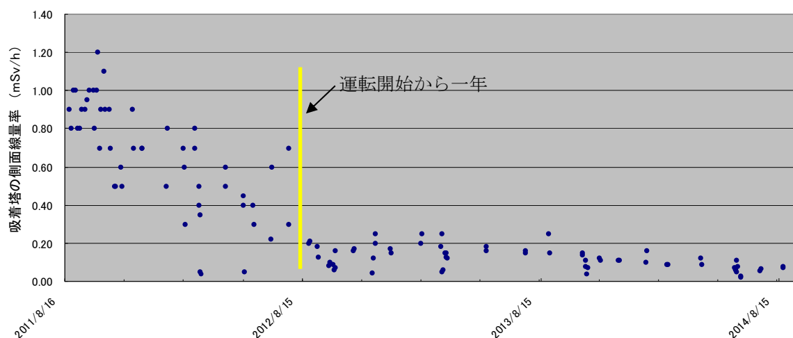
図 3 一時保管施設に保管した第二セシウム吸着装置吸着塔の発生時期と側面線量率分布
