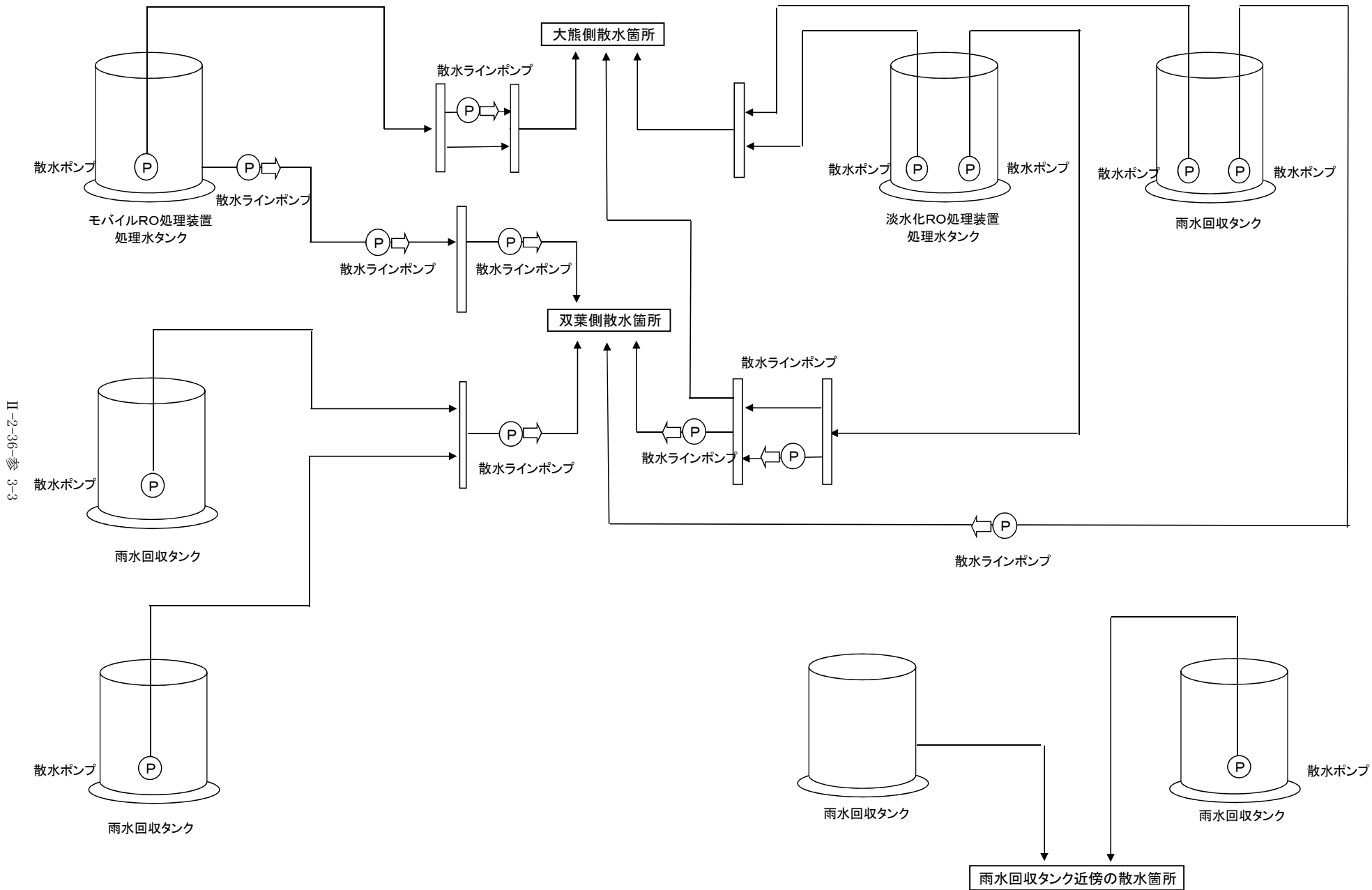
図ー1 散水設備概略図
