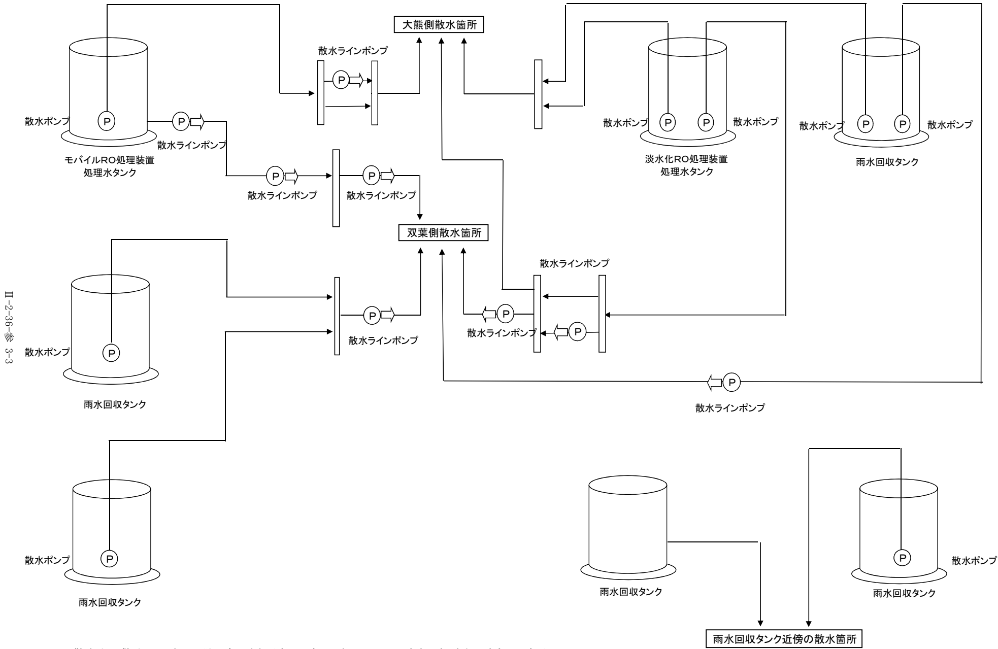
図-1 散水設備概略図
