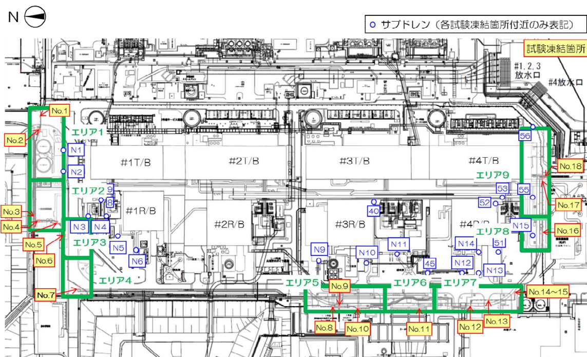
図1 試験凍結箇所付近のサブドレン位置図
