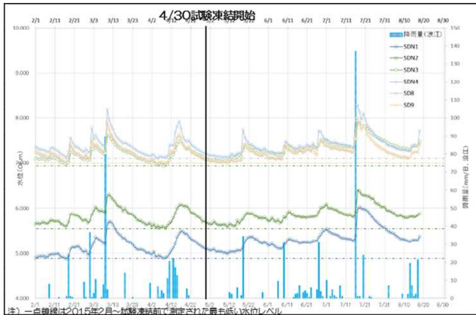
図2-1 サブドレン水位の経時変化 (エリア1・2付近)
