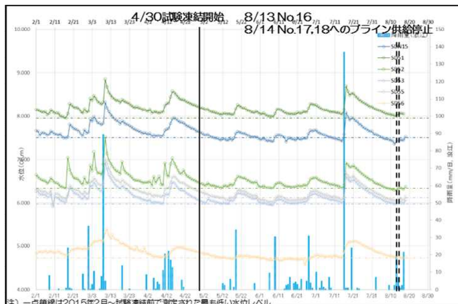
図2-6 サブドレン水位の経時変化 (エリア8・9付近)
