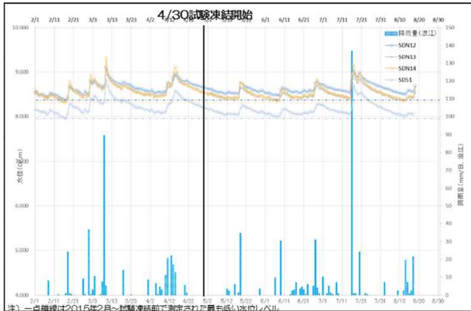
図2-5 サブドレン水位の経時変化 (エリア7付近)
