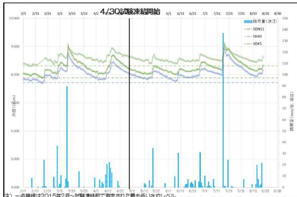
図2-4 サブドレン水位の経時変化 (エリア 6 付近)
