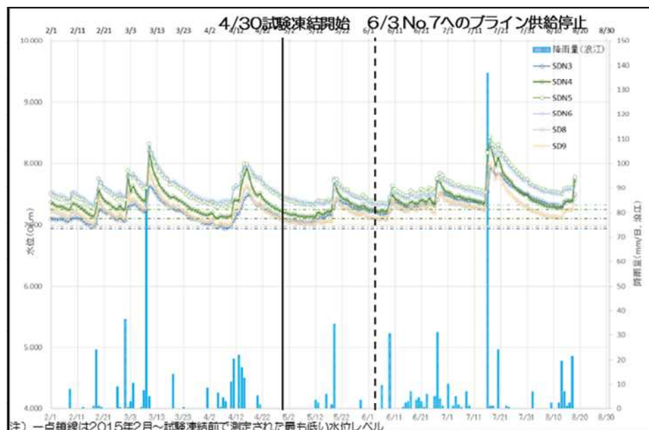
図2-2 サブドレン水位の経時変化 (エリア3・4付近)
