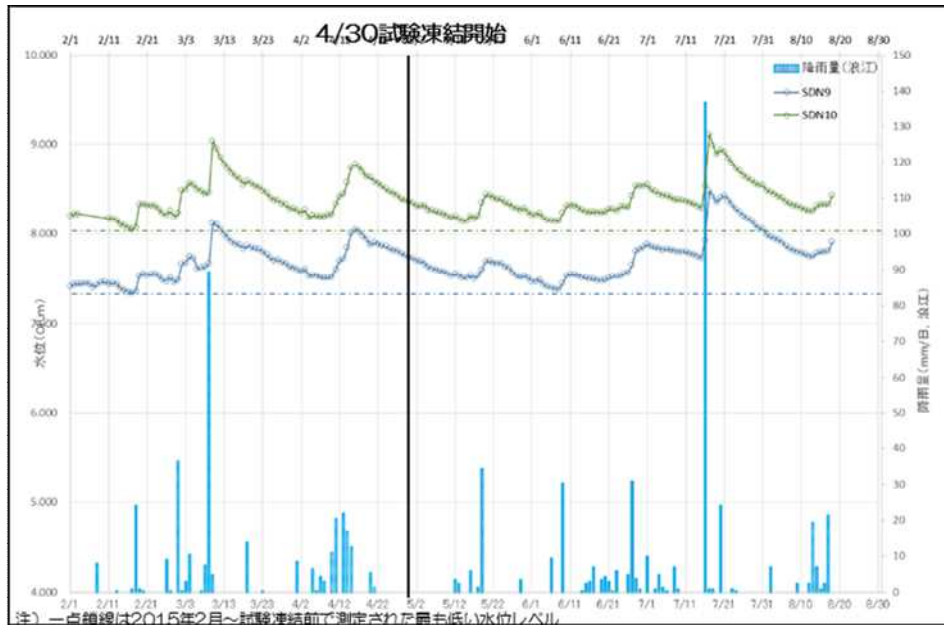
図2-3 サブドレン水位の経時変化 (エリア 5 付近)
