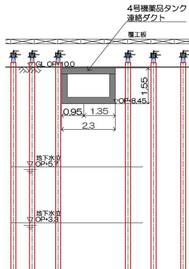
断面図
