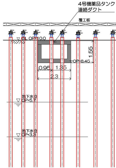
断面図
