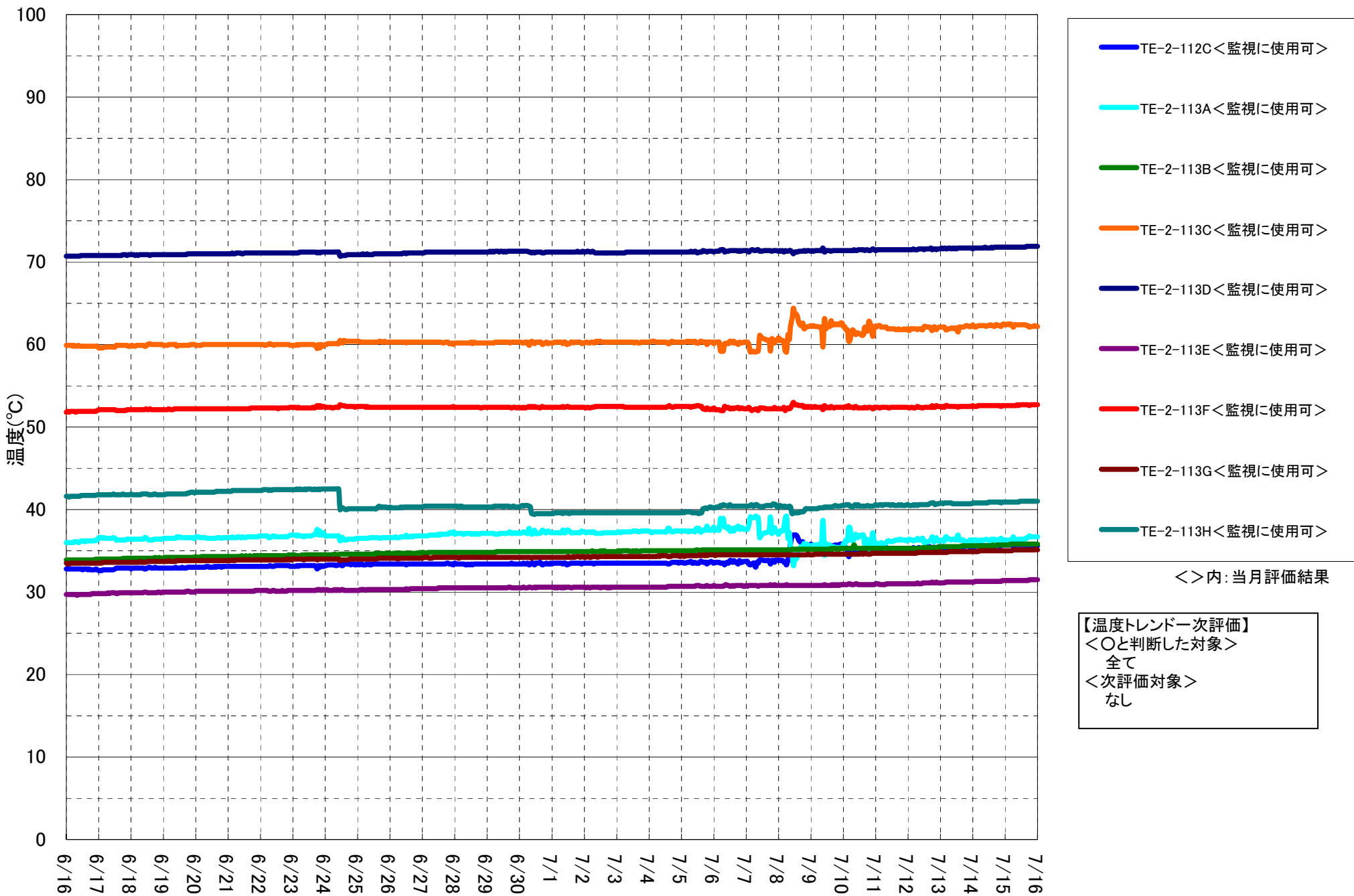
2号機 PCV内温度計①
