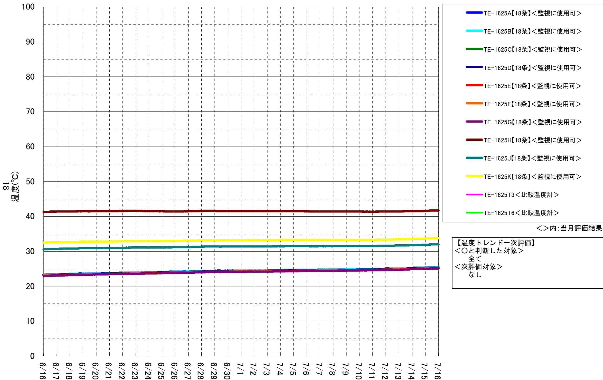
1号機 実施計画関連温度計(PCV)
