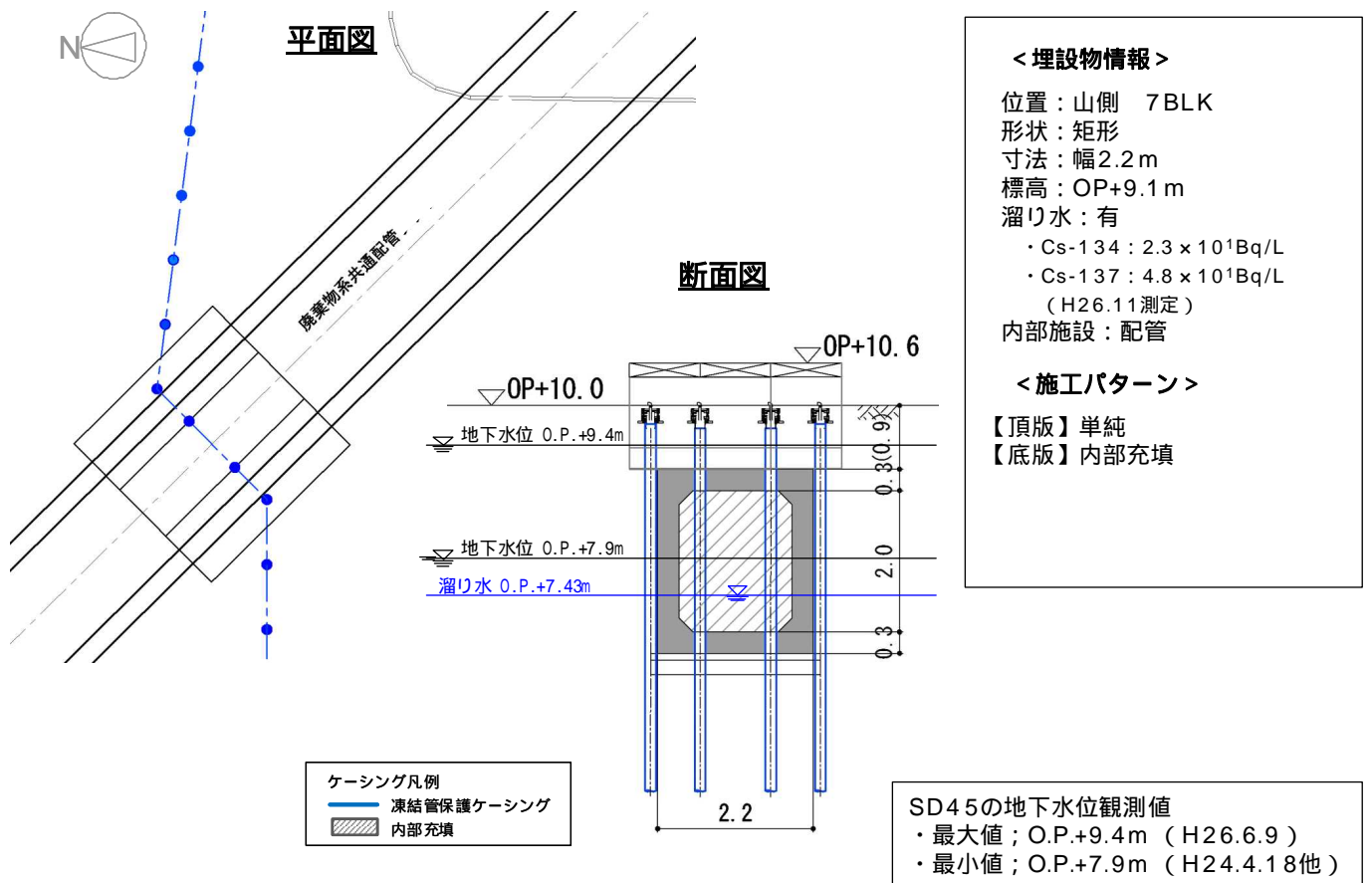
図 16 - 23 【7 - 5】廃棄物系共通配管ダクト 施工方法（貫通施工）
