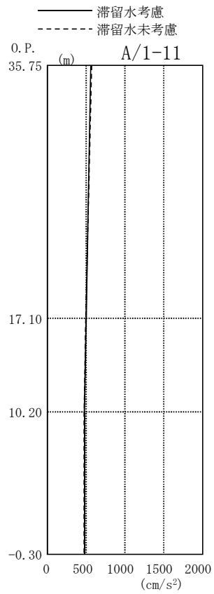
图 3.1.5-1 最大応答加速度 (NS 方向・S S -1H)
