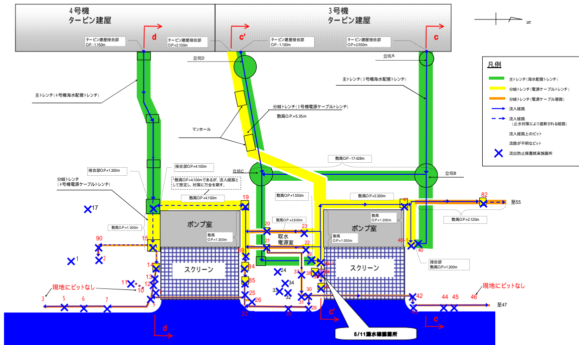
図4 3 / 4号機海側側トレンチ平面図
