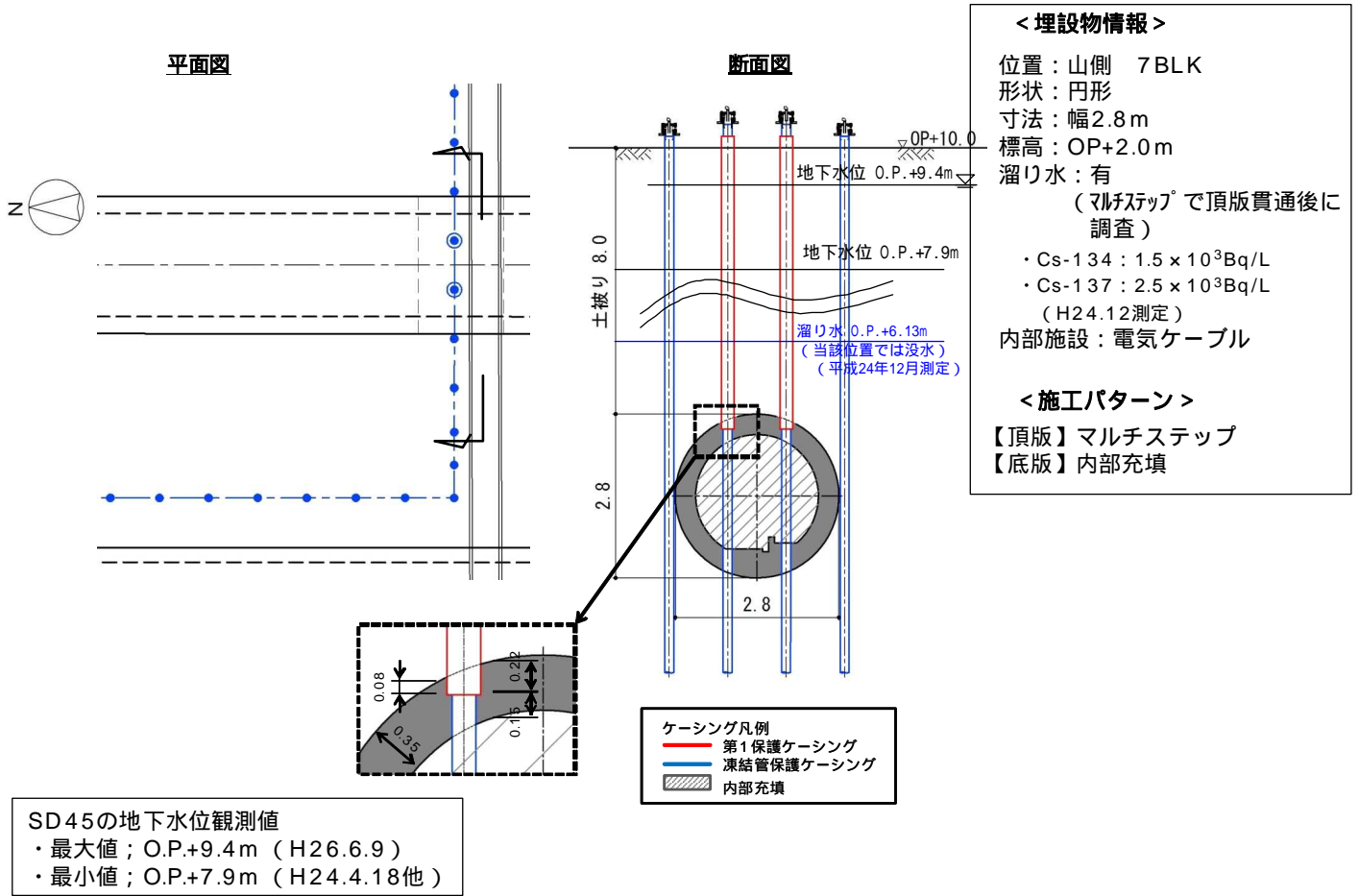
図16-19 【7-1】2~4号機DG連絡ダクト 施工方法（貫通施工）
