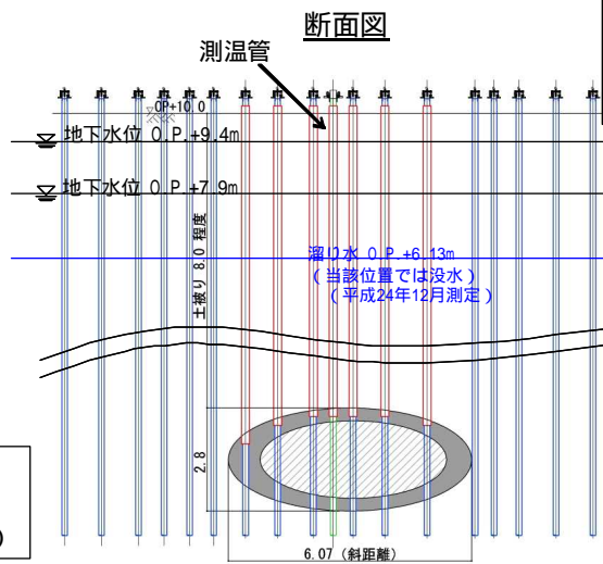
図16-20 【7-2】2~4号機 DG 連絡ダクト 施工方法 (貫通施工)
