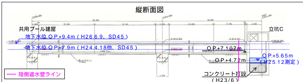
図16-17 【6-8】2~4号機DG連絡ダクト 施工方法(貫通施工)
