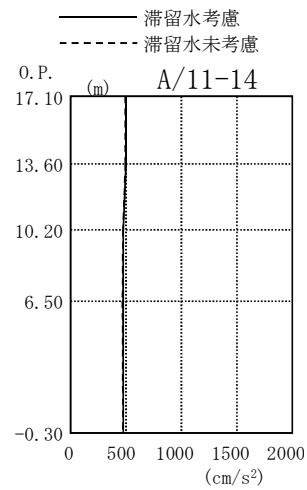
图 3.1.5-1 最大応答加速度 (NS 方向・S S -1H)
