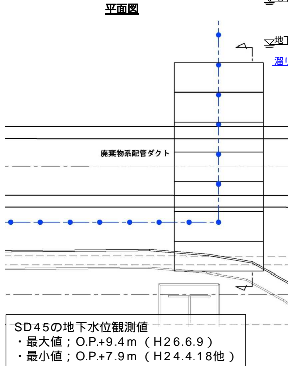
図16-22 【7-4】廃棄物系共通配管ダクト 施工方法(貫通施工)
