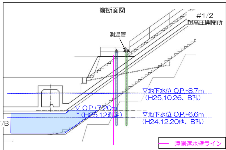
図16-8 【5-1】1号機電気ケーブルダクト 施工方法（貫通施工）
