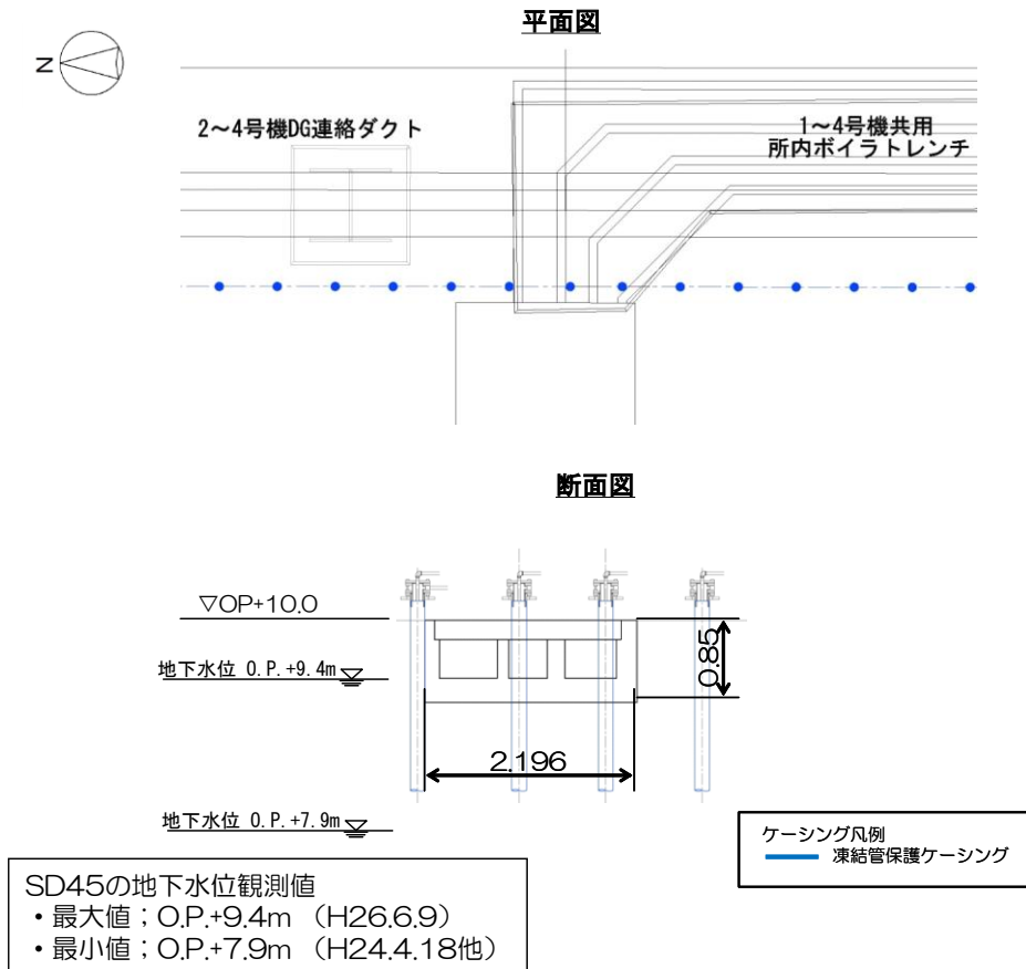
図 1 6 - 1 3 【 6 - 4 】 1 ~ 4 号機共用所内ボイラトレンチ 施工方法（貫通施工）
