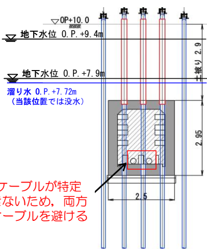
断面図
