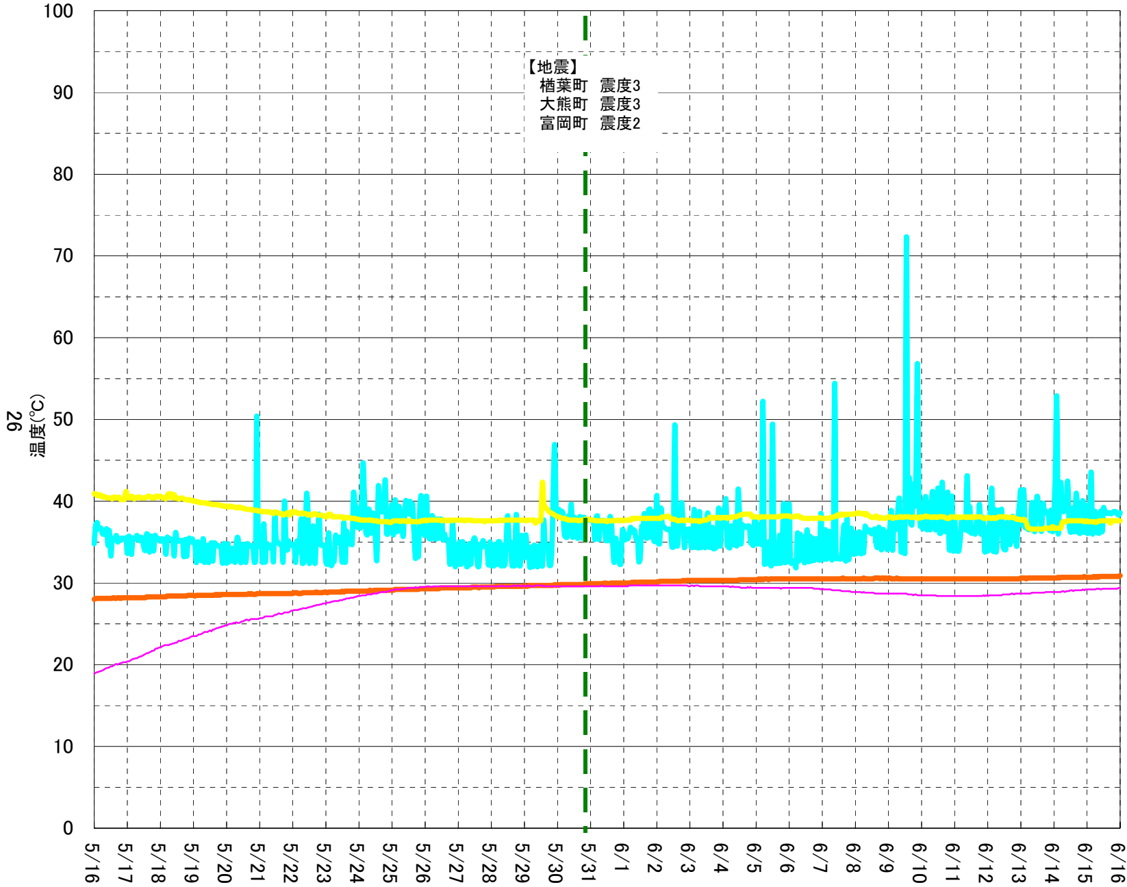
2号機 RPV周辺温度計(下部)
