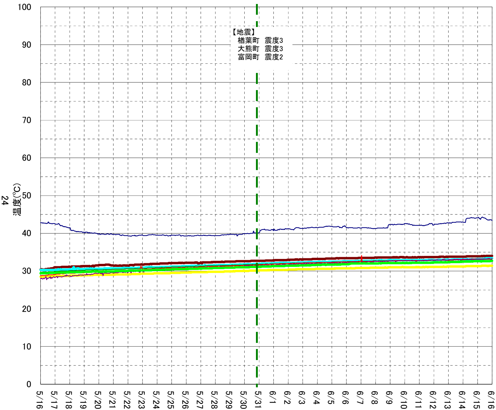
2号機 RPV周辺温度計(上部)①
