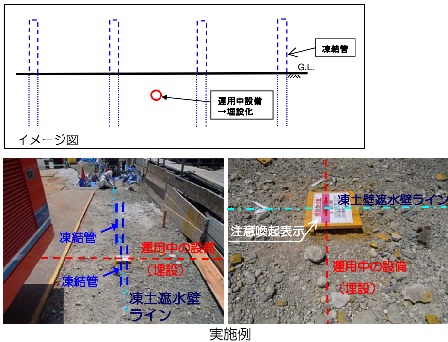
図9-2 運用中の設備の防護パターンB
