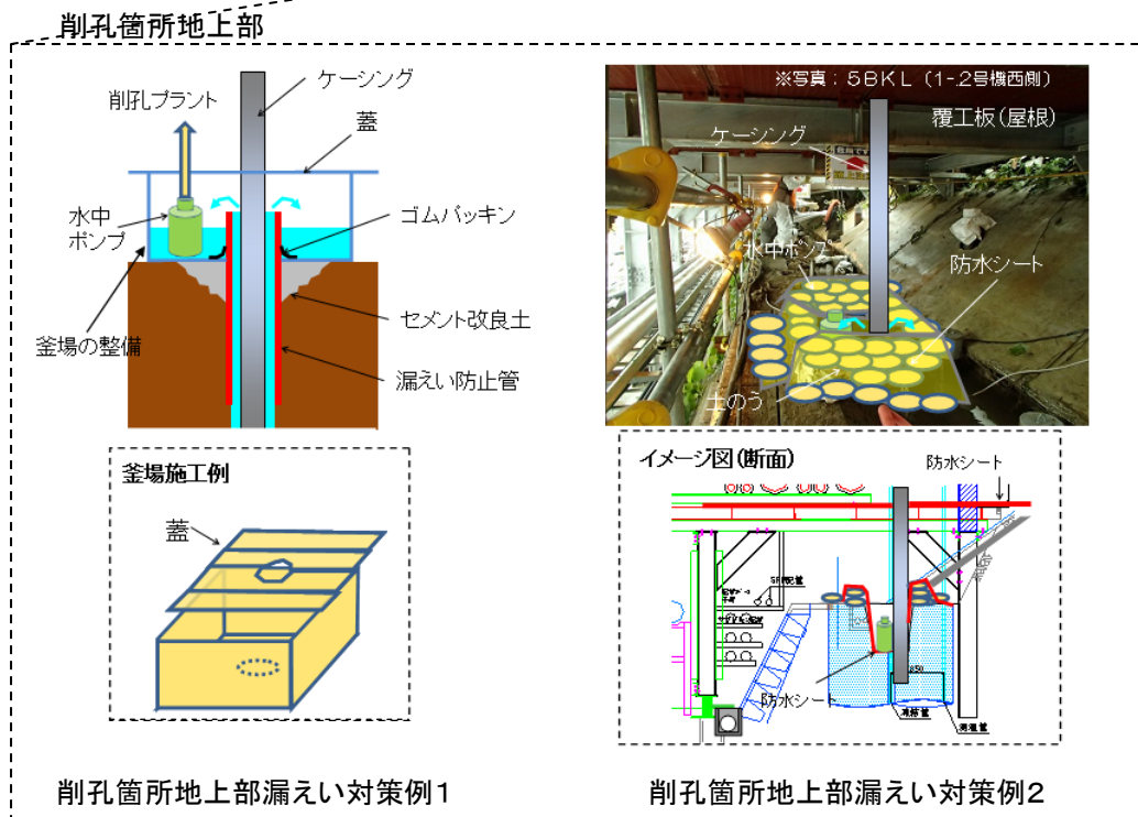
図 1 1 削孔水の漏えい対策イメージ
