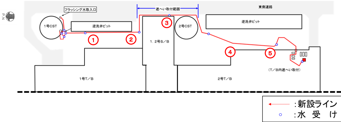
図3 移送ラインの敷設ルート（新設ライン）
