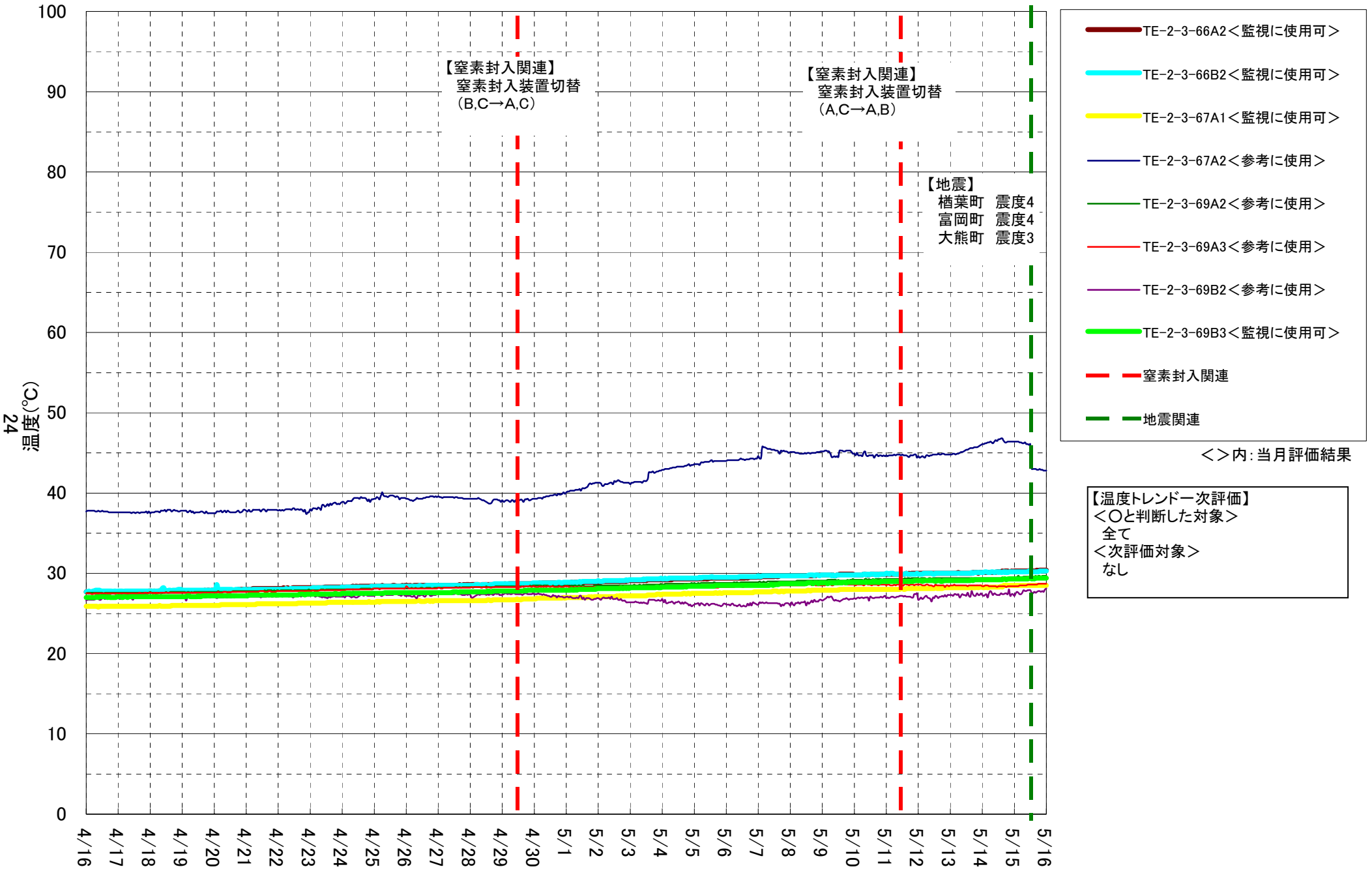
2号機 RPV周辺温度計(上部)①
