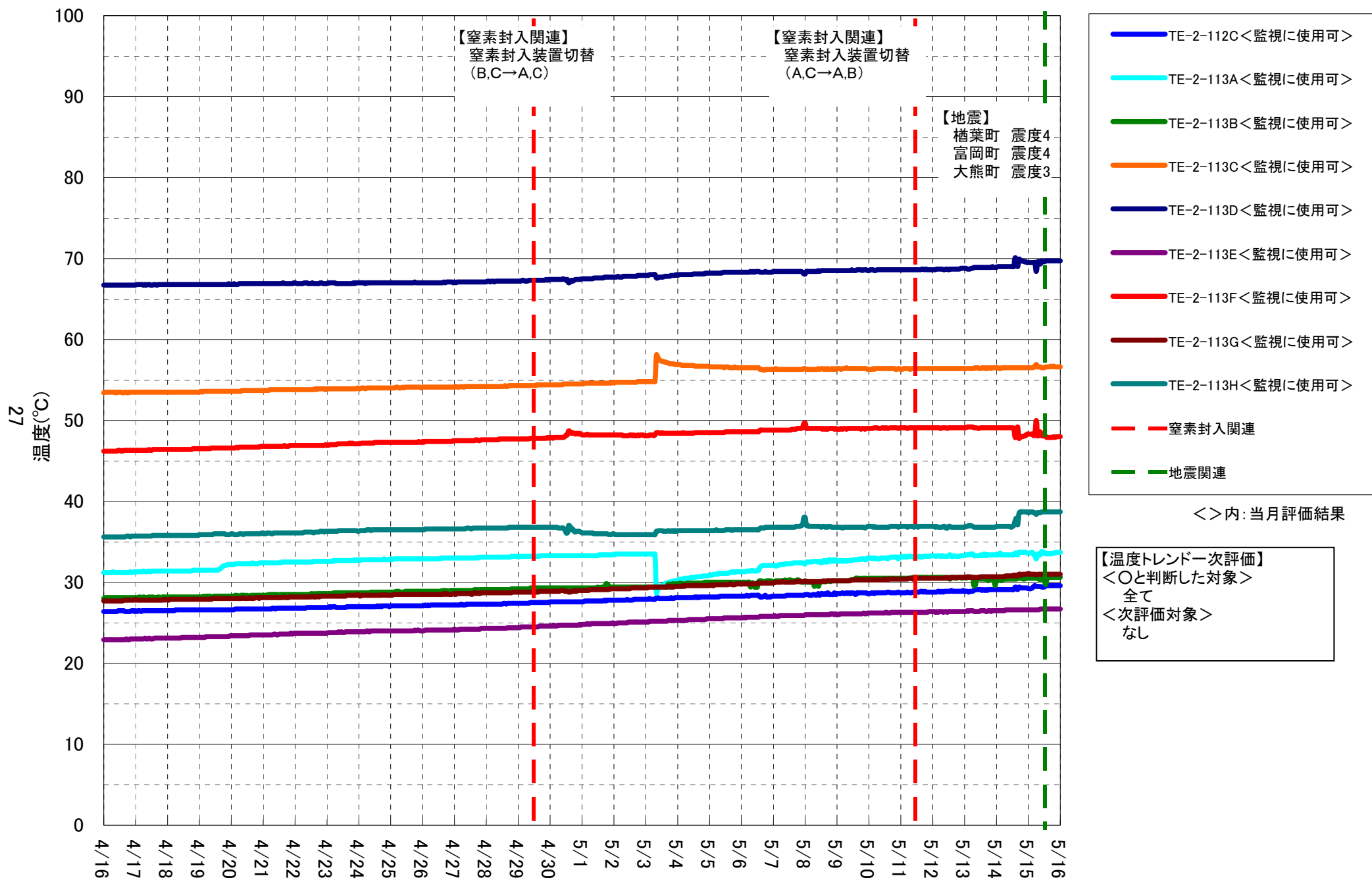
2号機 PCV内温度計①
