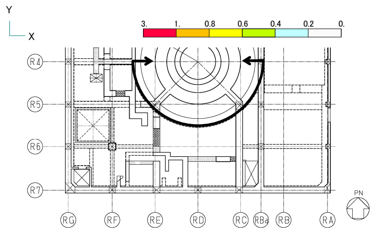
図-12 面外せん断力の検定比 (シェル壁部)
