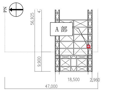
キープラン (O.P. 46.000 伏図)
