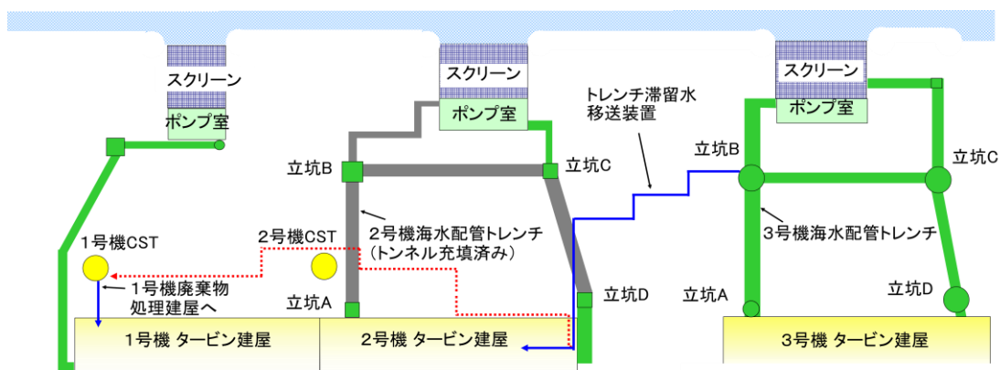
図-1 トレンチからCSTの移送ライン
