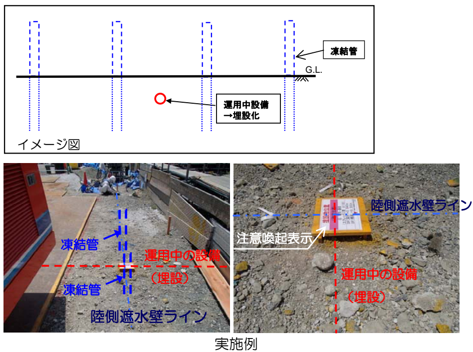
図9-2 運用中の設備の防護パターンB
