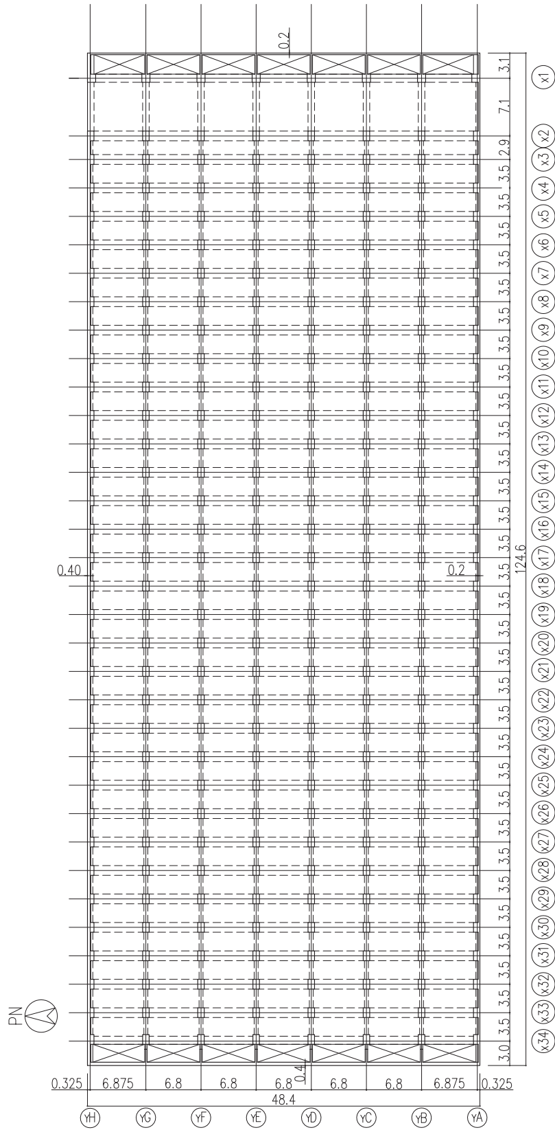
图一 5 地上2階平面図 (G.L.+4.7) (单位:m)
