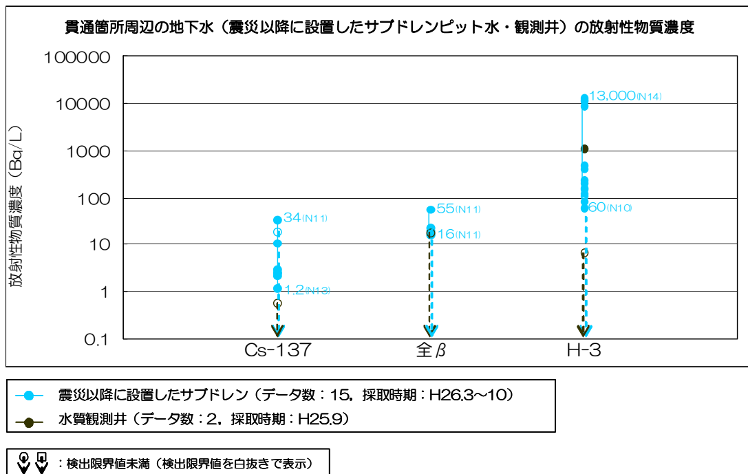
図 1 5 埋設物内に溜り水を有する貫通箇所周辺の地下水（サブドレンピット・観測井）の放射性物質濃度分布
