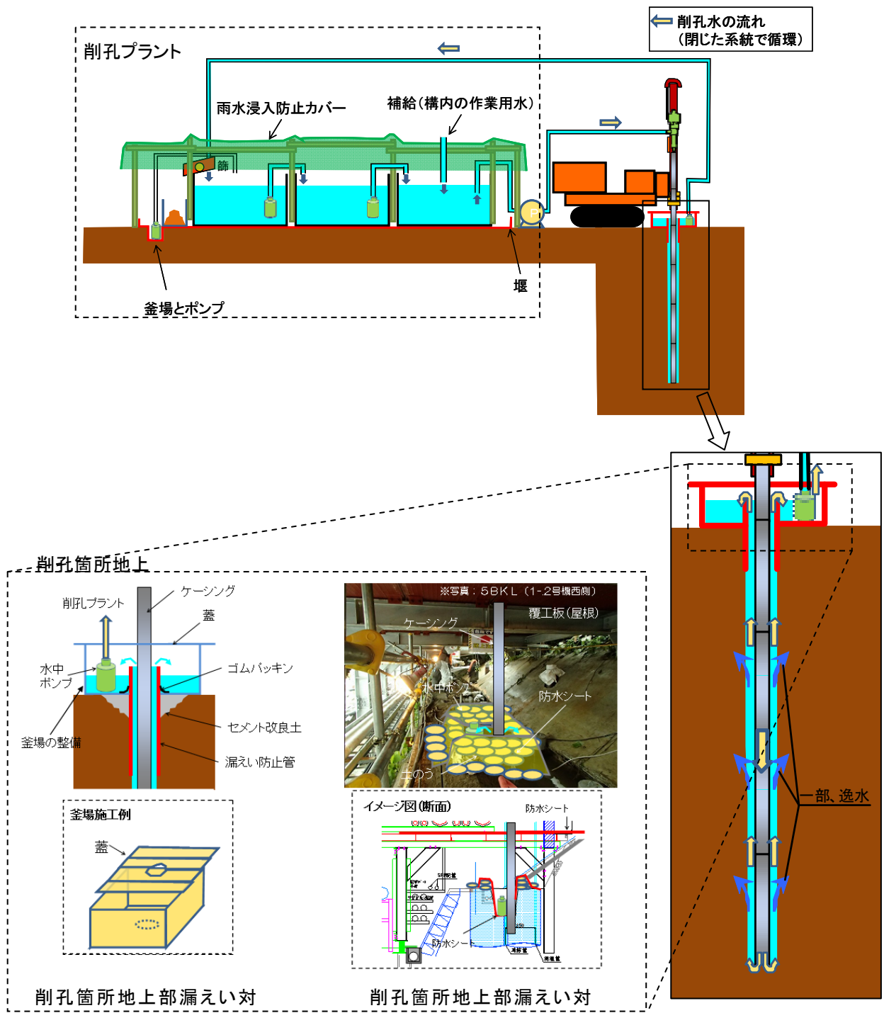
図 1 3 - 1 削孔水の漏えい対策イメージ (既認可)
