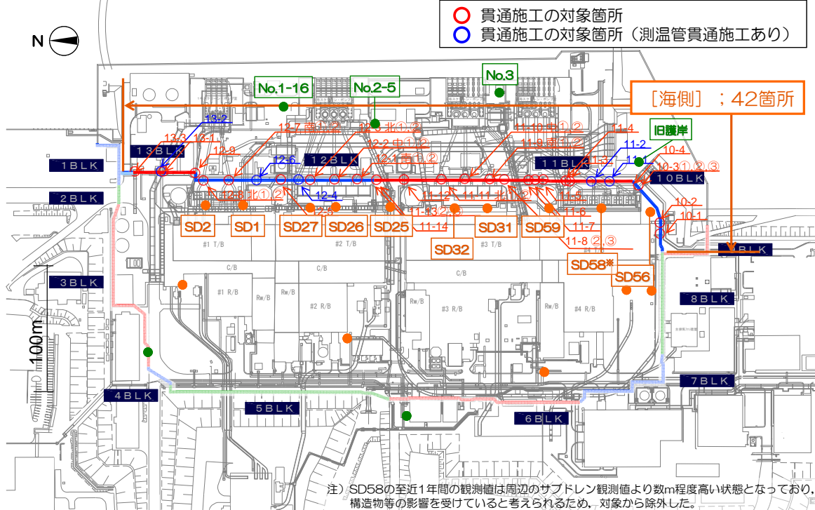
図 7-31 陸側遮水壁ライン近傍のサブドレン・地下水位観測孔 配置図
