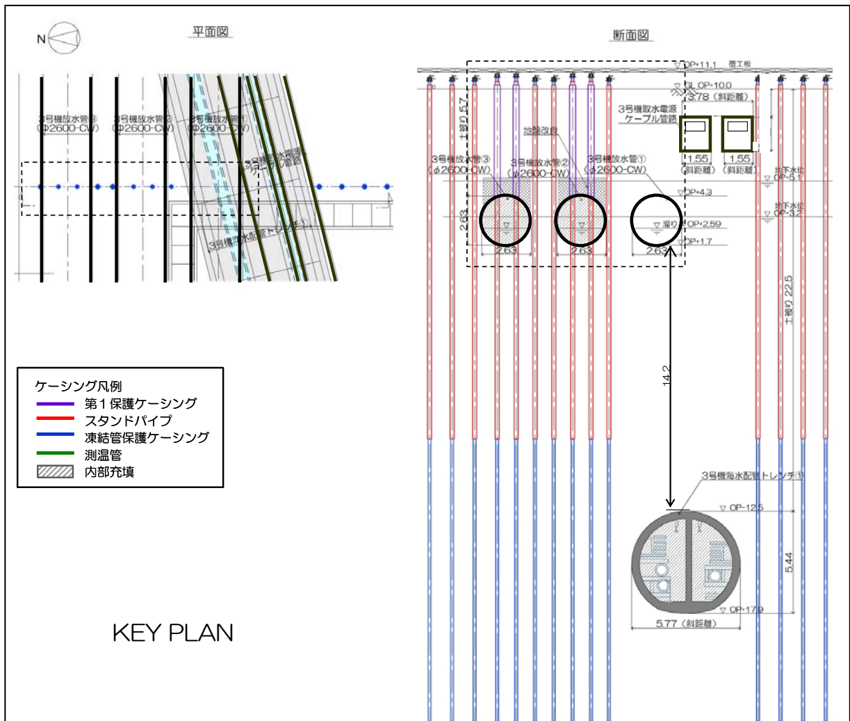
図7-12 【11-8】3号機放水管②③ 施工方法（貫通施工）
