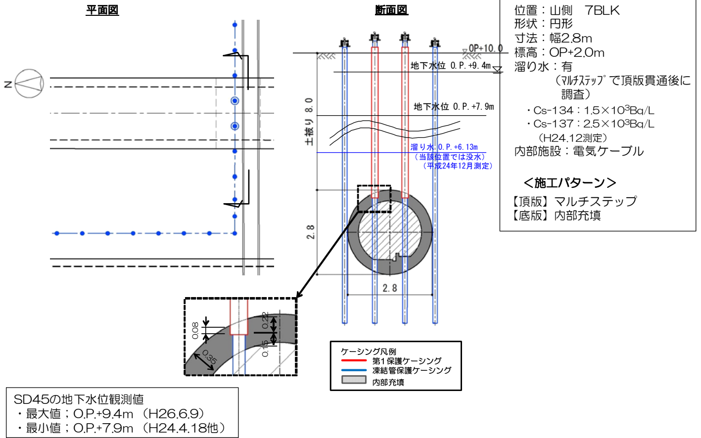
図14-18 【7-1】2~4号機DG連絡ダクト② 施工方法 (貫通施工)
