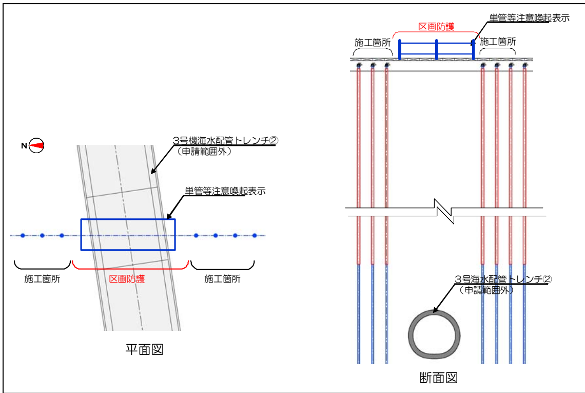
図 1 1 - 3 申請対象外の区画防護 c
