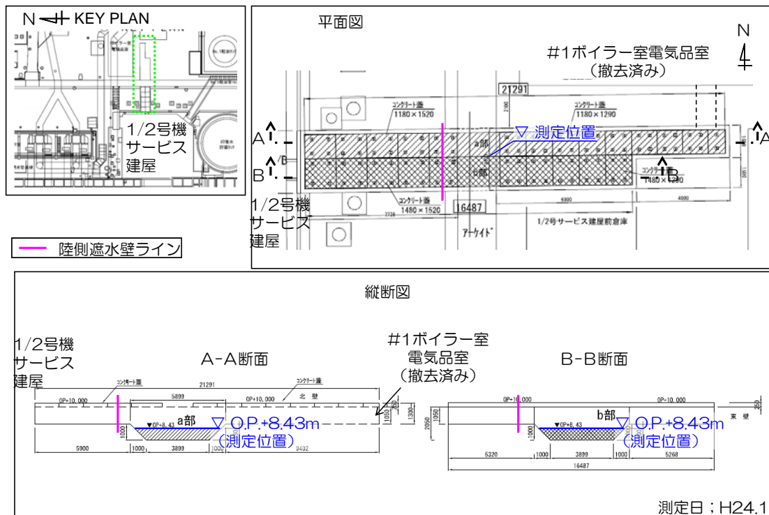
図7-24 【12-6】1号機ボイラー室電気品室連絡トレンチ 施工方法（貫通施工）
