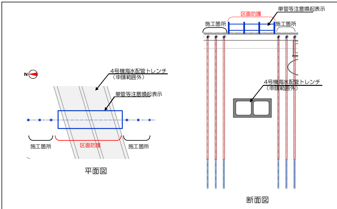
図 1 1 - 1 申請対象外の区画防護 a
