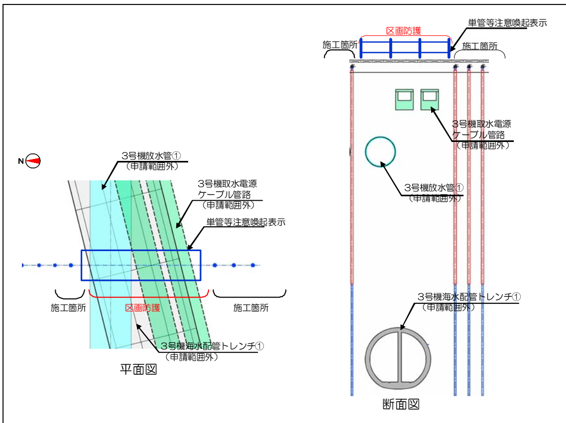
図 1 1 - 2 申請対象外の区画防護 b
