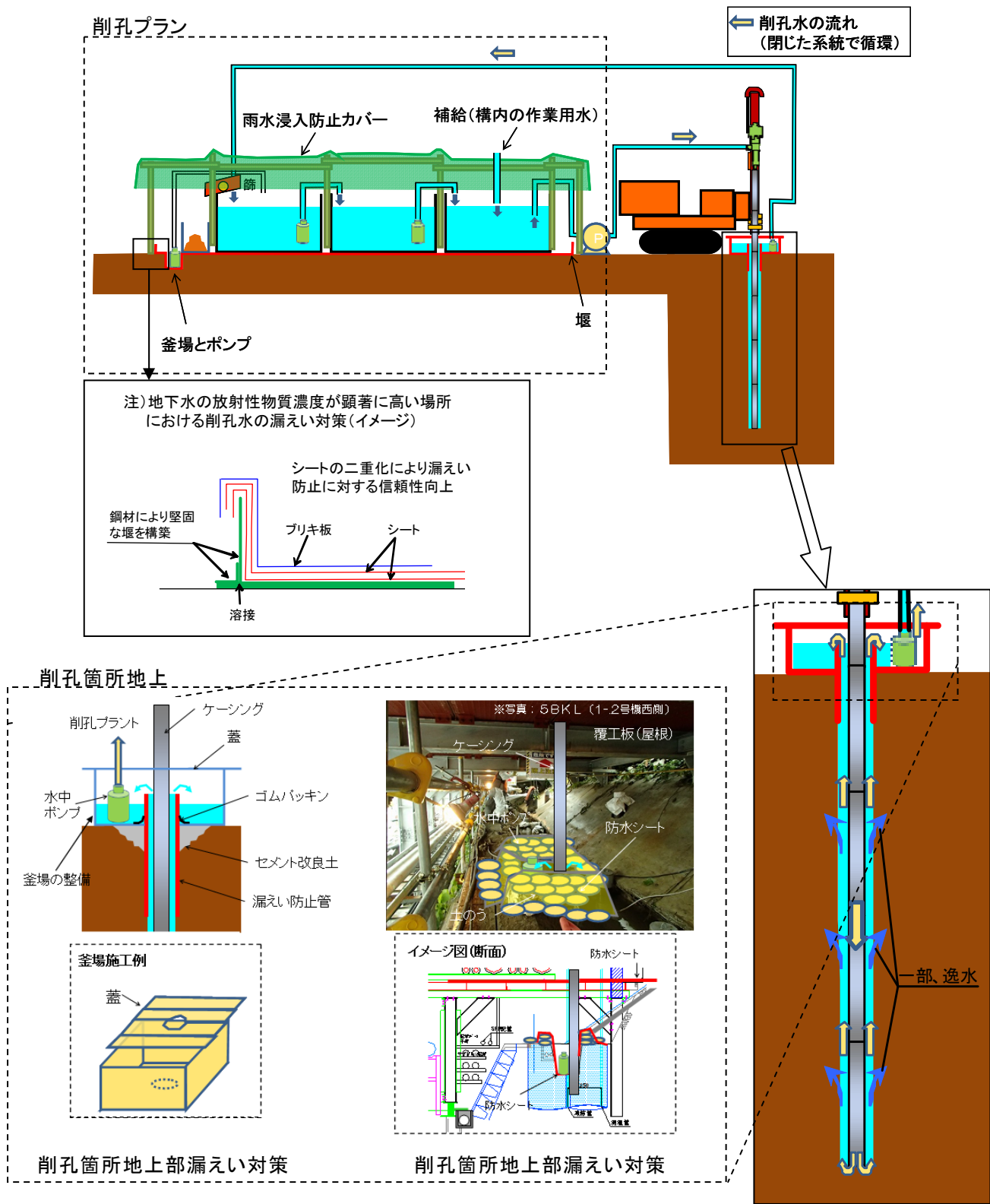
図13-2 削孔水の漏えい対策イメージ (今回申請)
