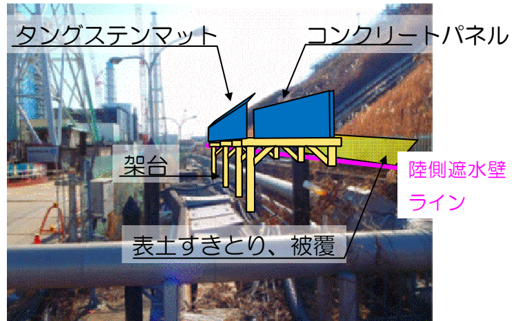
図 1 4 - 1 被ばく線量低減対策実施例 1 (既認可)
