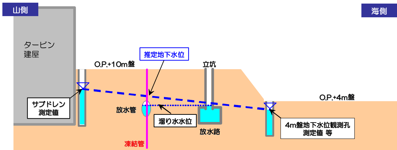
図5 貫通箇所における地下水位推定方法
