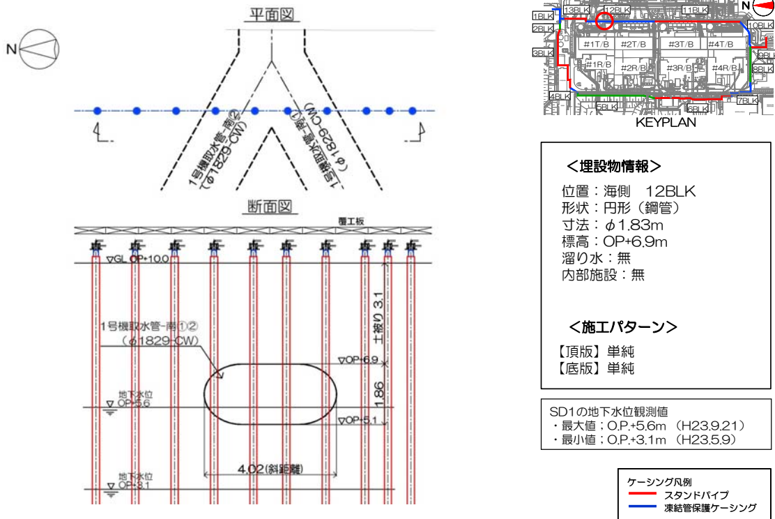
図 7-25 【12-7】1号機取水-南①② 施工方法（貫通施工）
