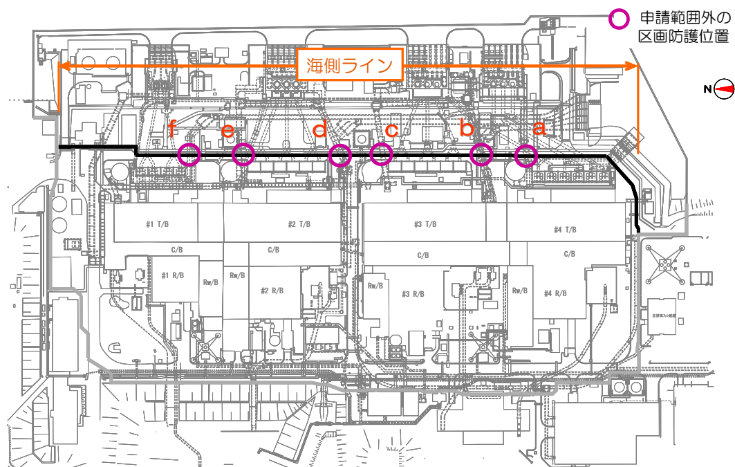
図 10 申請対象外の区画防護位置
