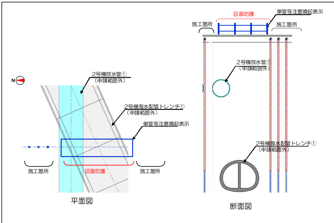
図 1 1 - 4 申請対象外の区画防護 d
