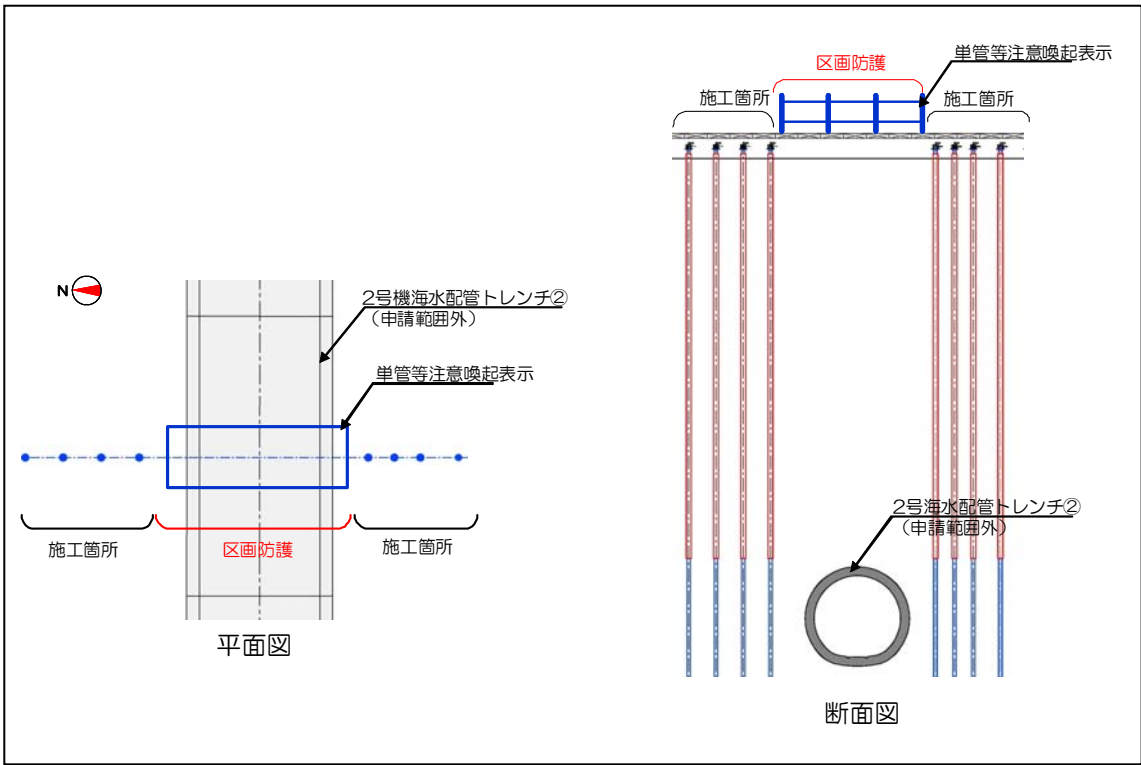
図 1 1 - 5 申請対象外の区画防護 e
