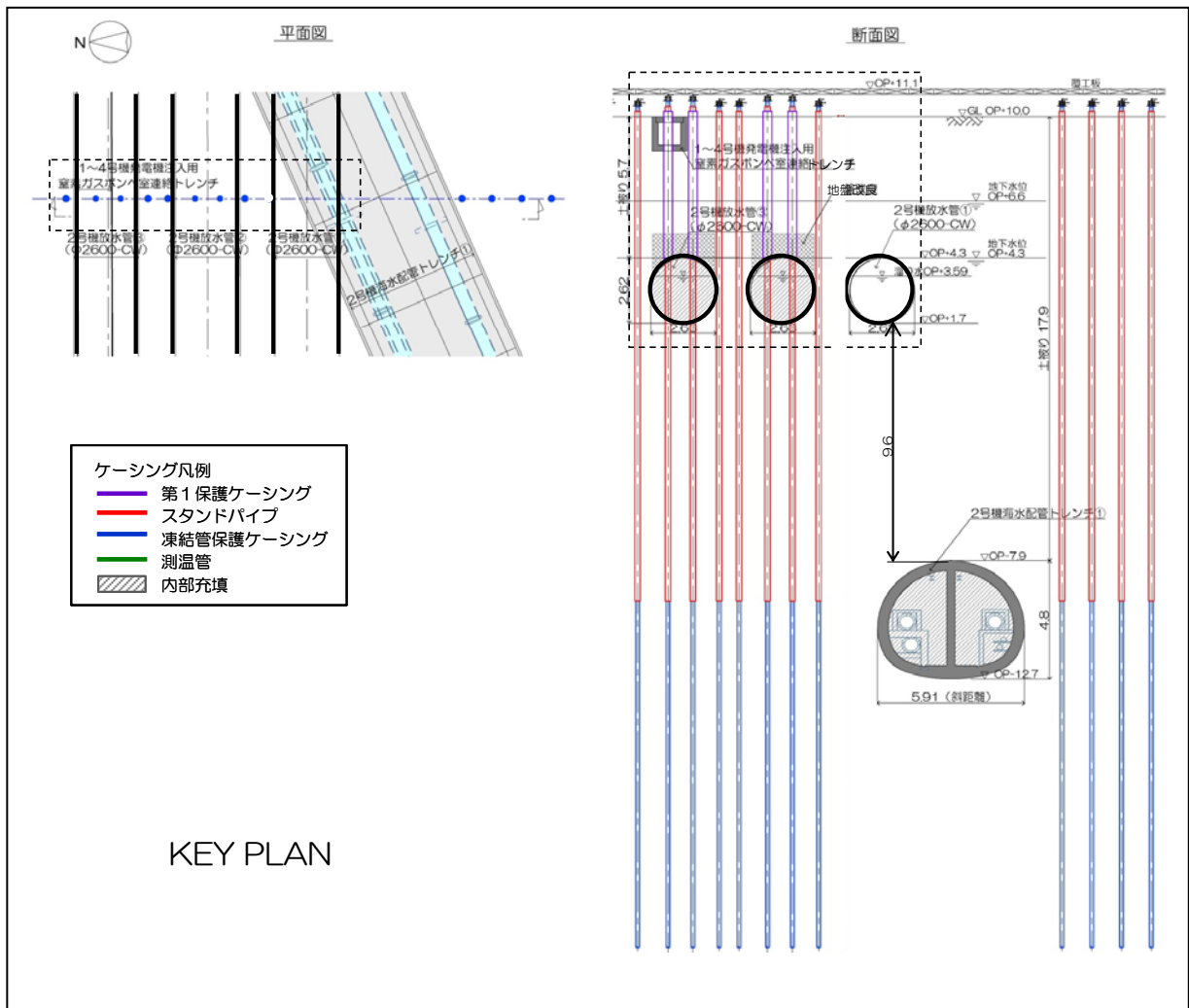
図7-17 【11-13】2号機放水管②③ 施工方法（貫通施工）
