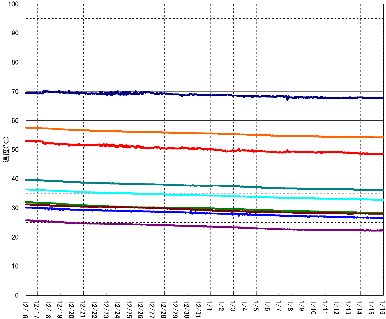
2号機 PCV内温度計①
