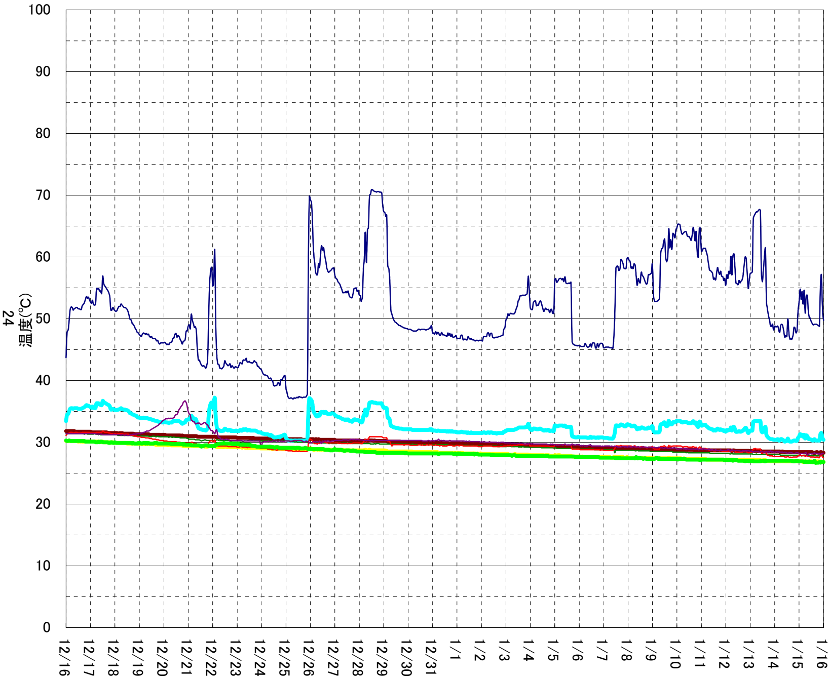
2号機 RPV周辺温度計(上部)①
