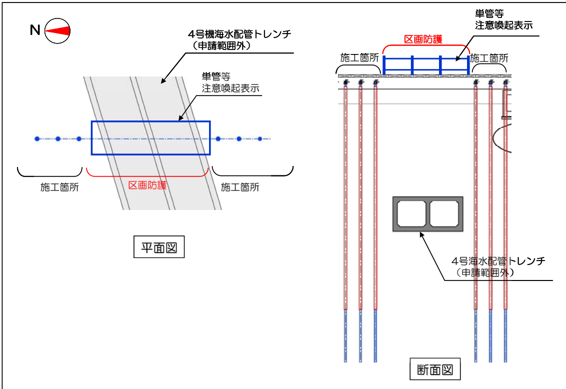
図 1 1 - 1 申請対象外の区画防護 a
