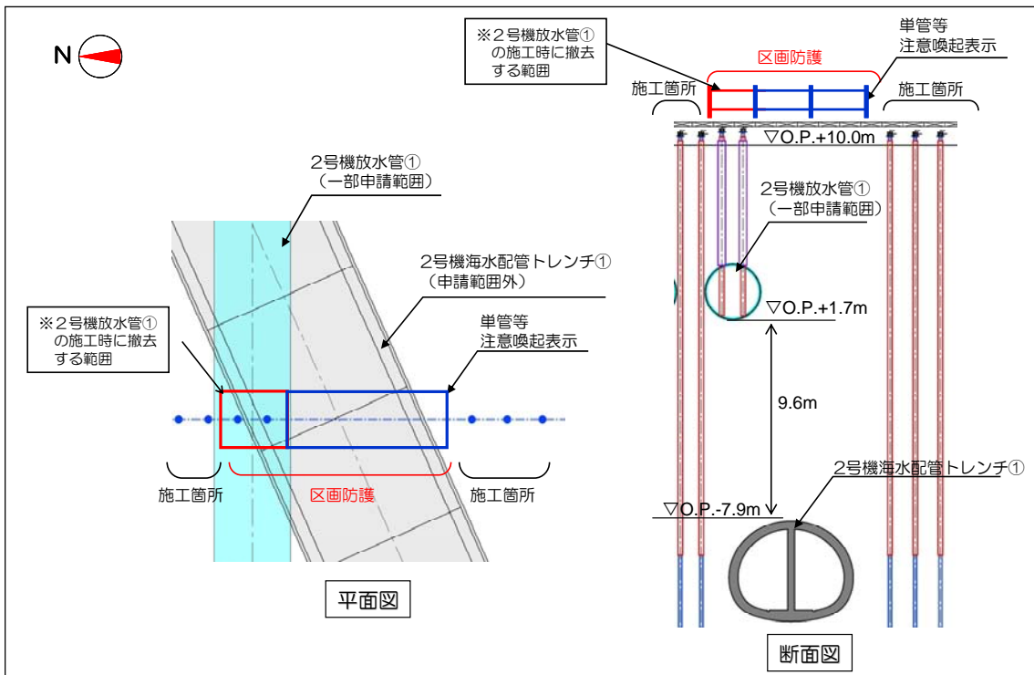
図 1 1 - 4 申請対象外の区画防護 d
