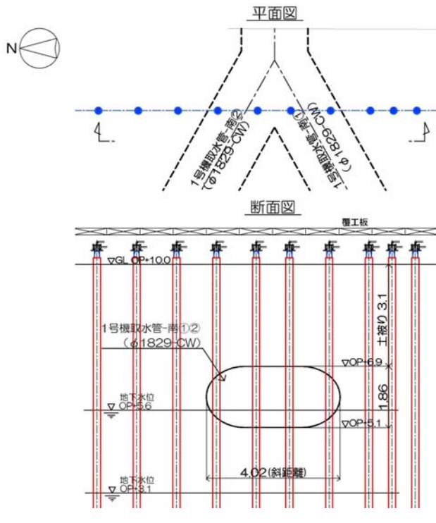
図 7-25 【12-7】1号機取水-南①② 施工方法（貫通施工）
