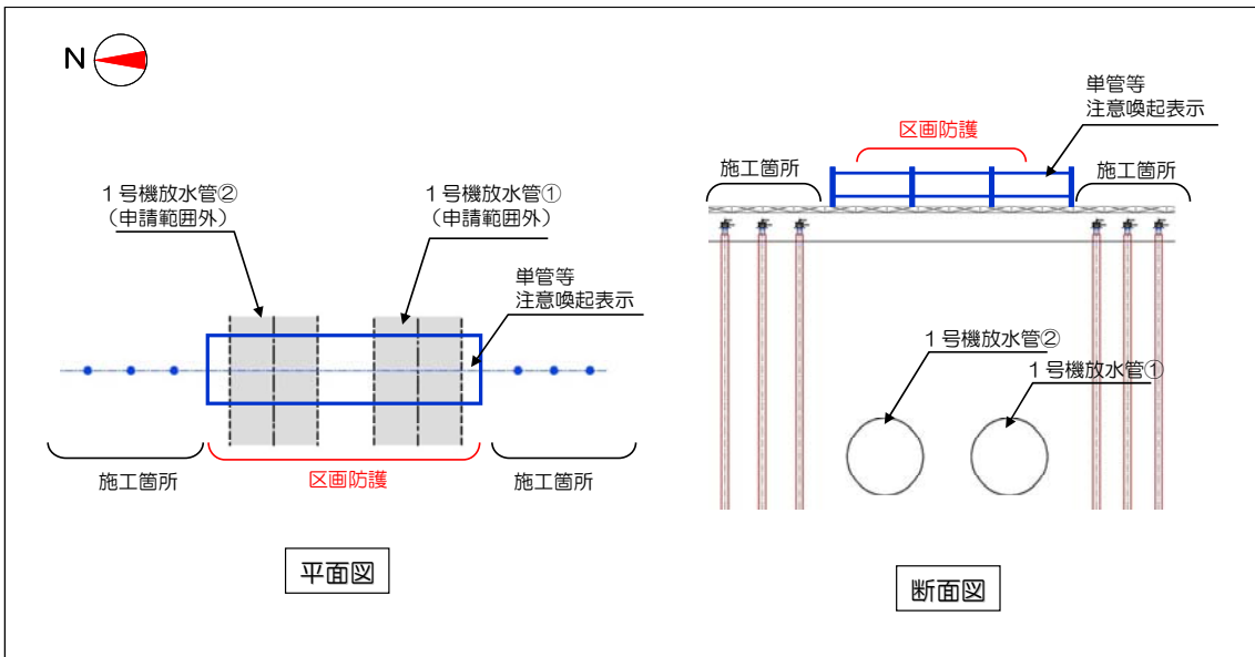
図 1 1 - 6 申請対象外の区画防護 f
