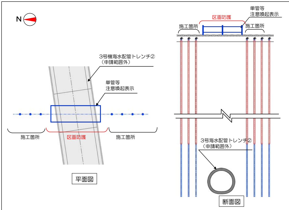
図 1 1 - 3 申請対象外の区画防護 c
