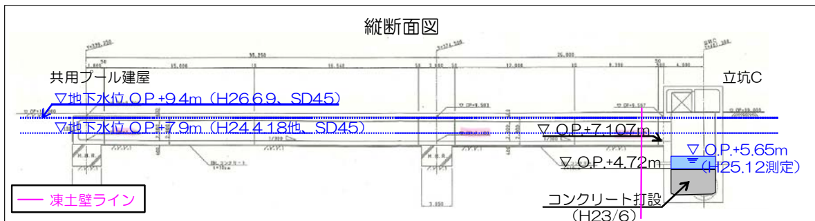
図14-16 【6-8】2~4号機DG連絡ダクト①施工方法（貫通施工）
