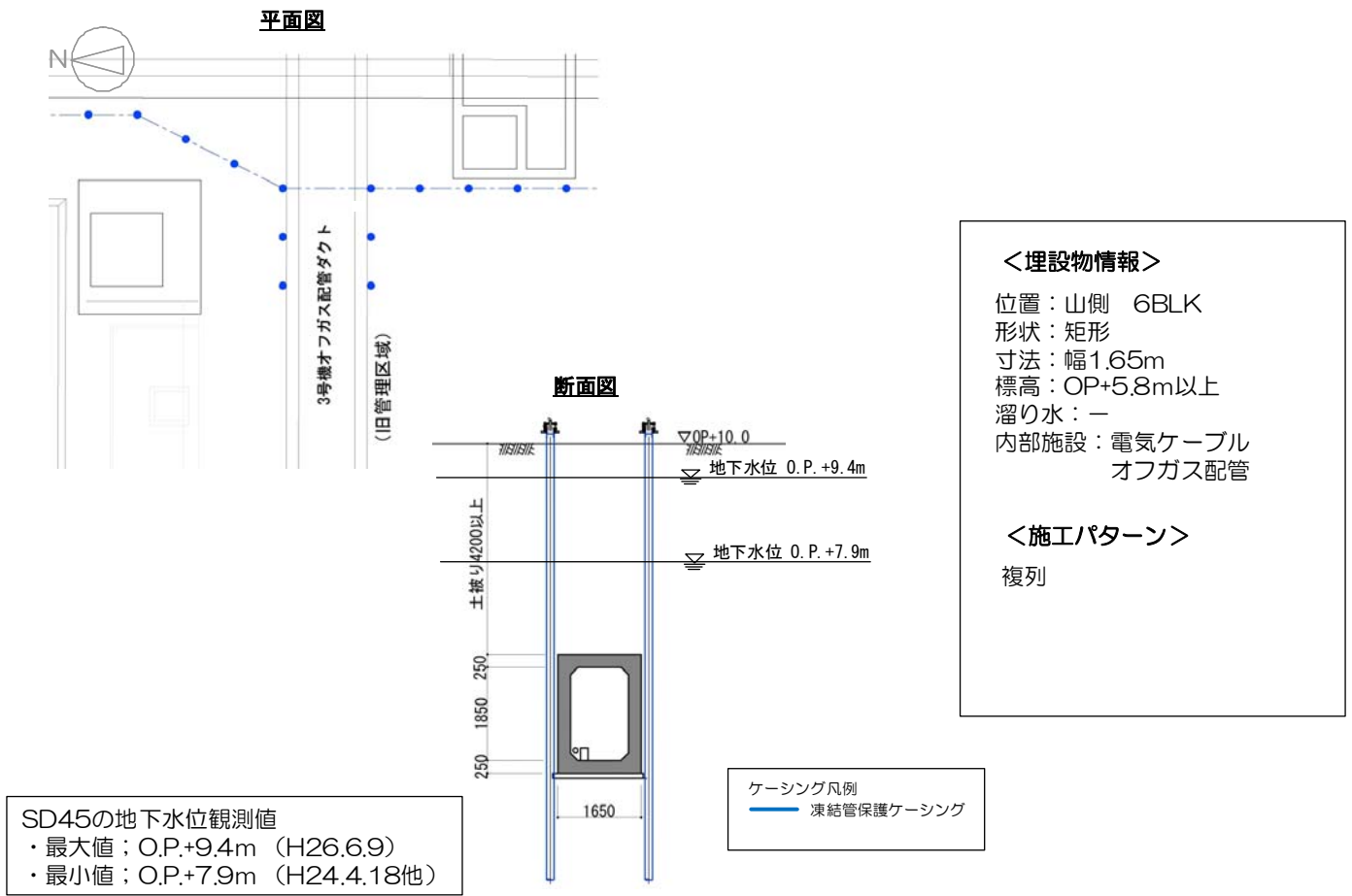
図14-11 【6-3】3号機オフガス配管ダクト（北側） 施工方法（複列施工）
