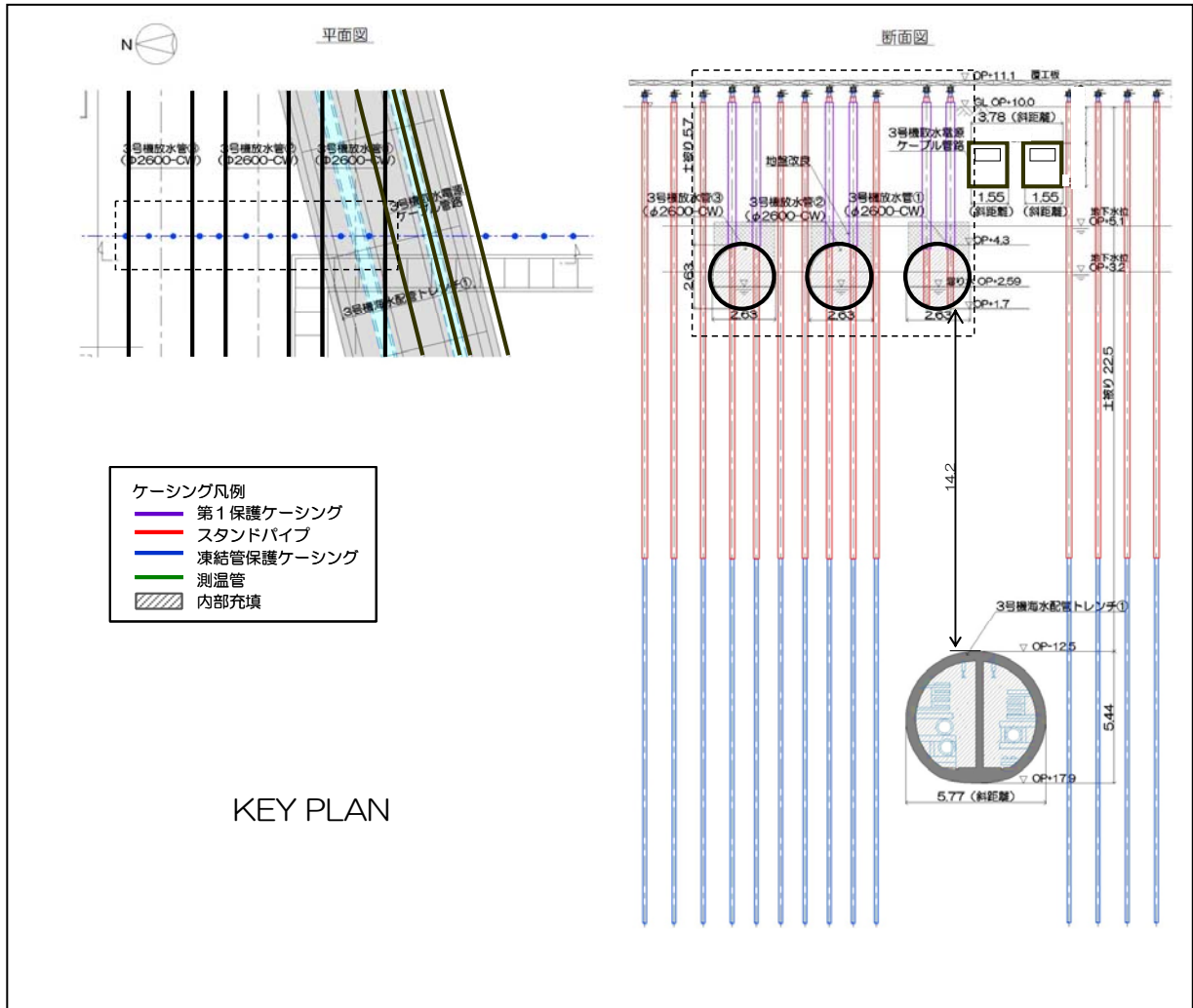
図7-12 【11-8】3号機放水水管①②③ 施工方法（貫通施工）
