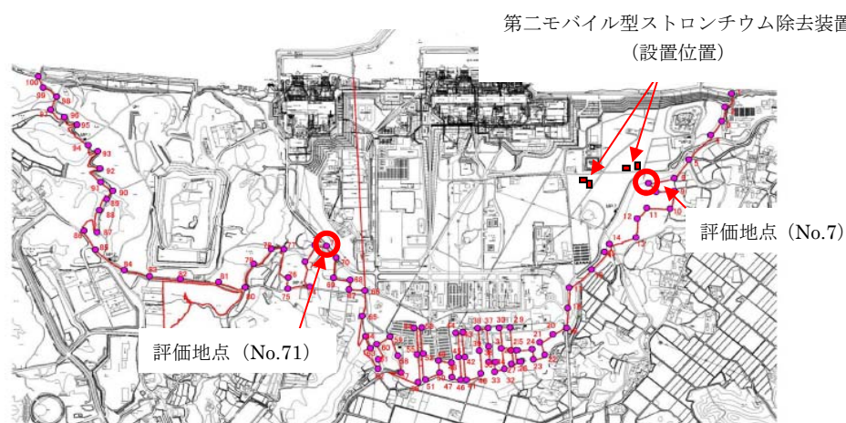
図-1 第二モバイル型ストロンチウム除去装置（当初設置位置）と評価点の位置関係
