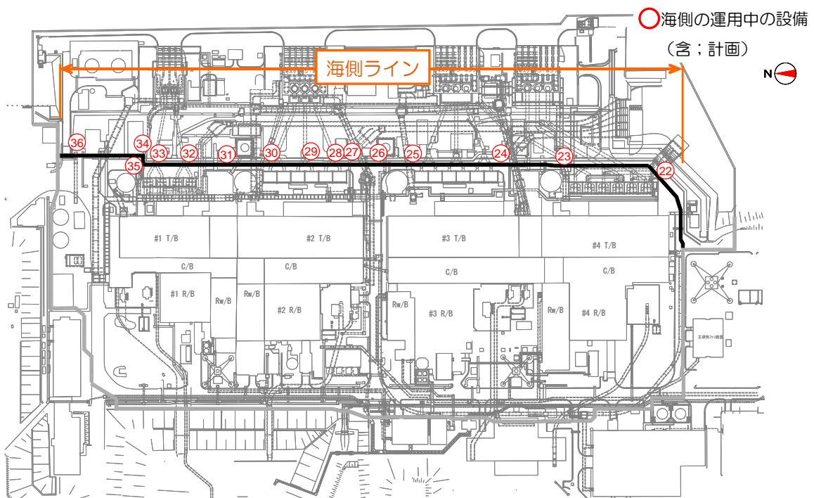
図 7 - 2 主な運用中の設備と凍土遮水壁の横断箇所（今回申請）
