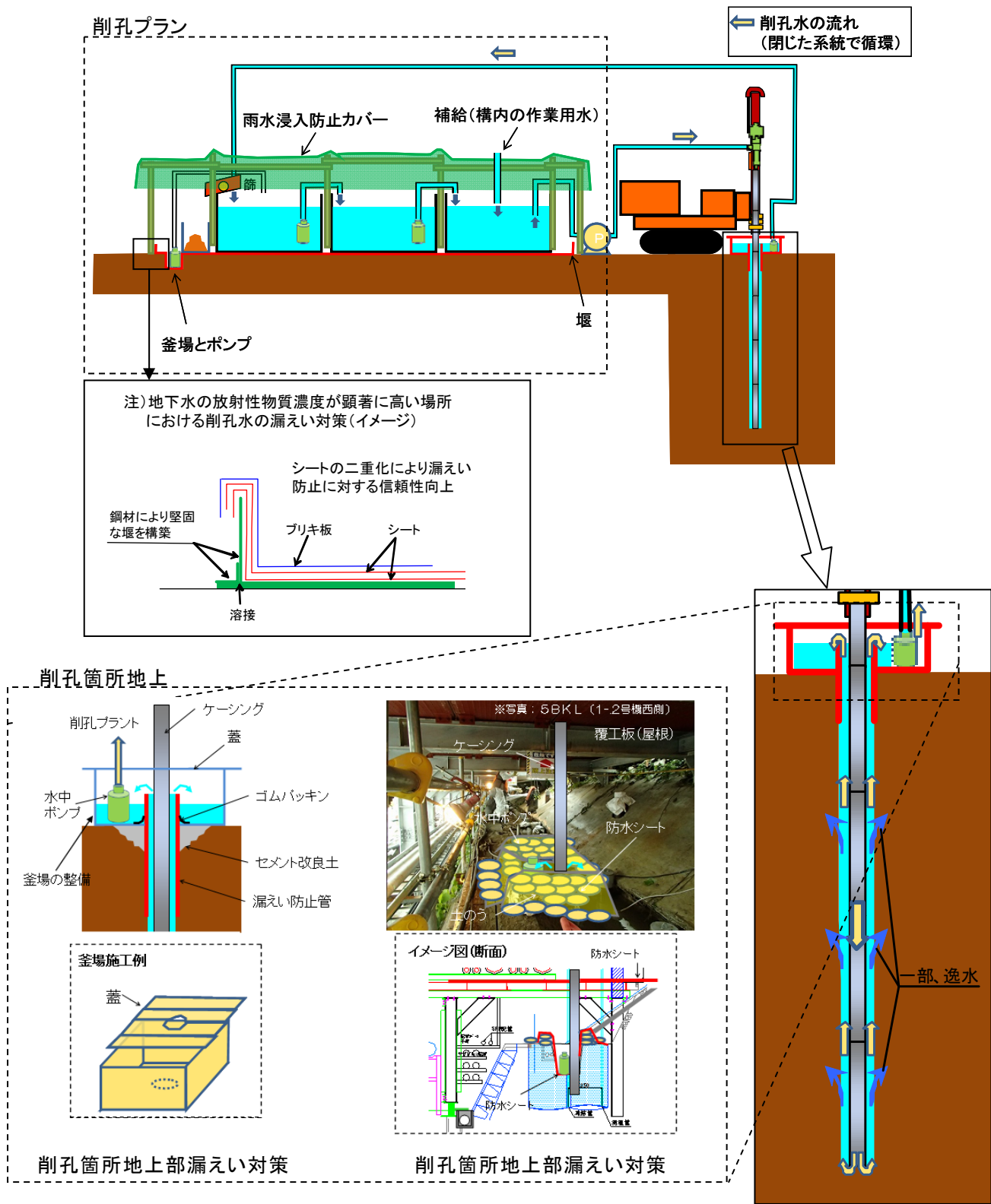
図 1 1 - 2 削孔水の漏えい対策イメージ (今回申請)
