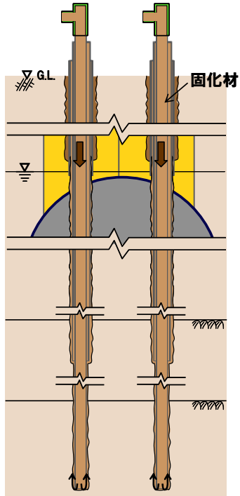
図3 頂版マルチステップ・底版内部充填工法の施工手順 (3)
