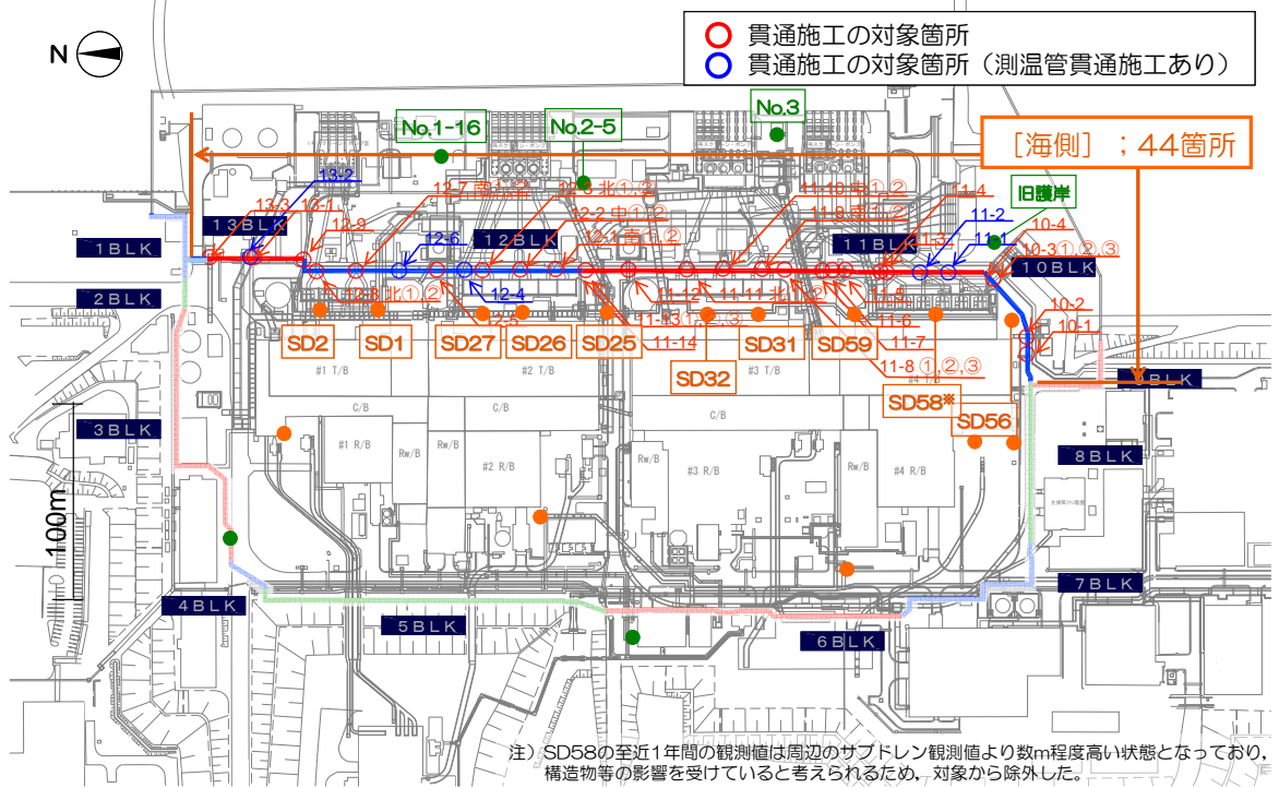
図 7 - 3 1 凍土壁ライン近傍のサブドレン・地下水位観測孔 配置図
