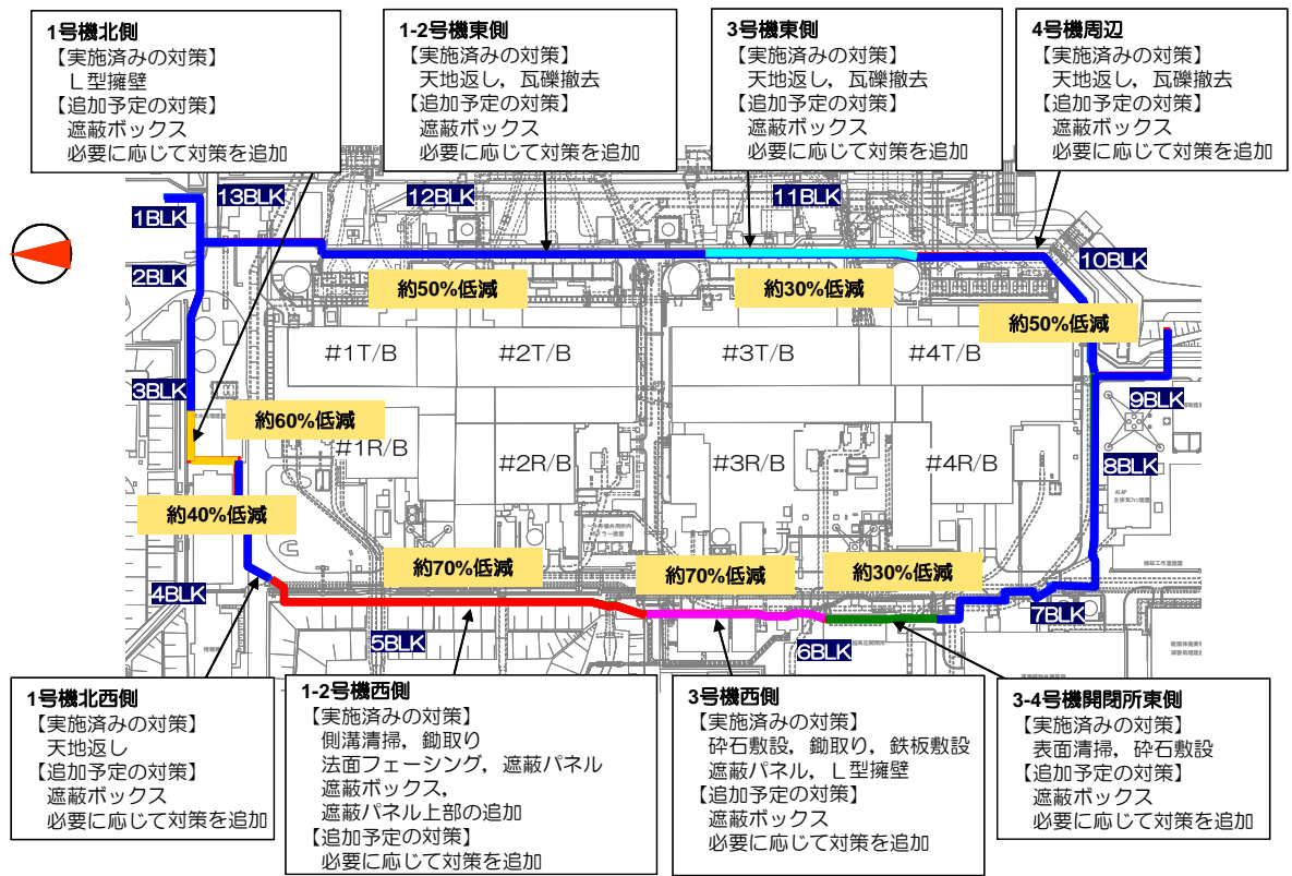
図 1 2 - 1 1 被ばく線量低減対策の実施状況 (今回申請)
