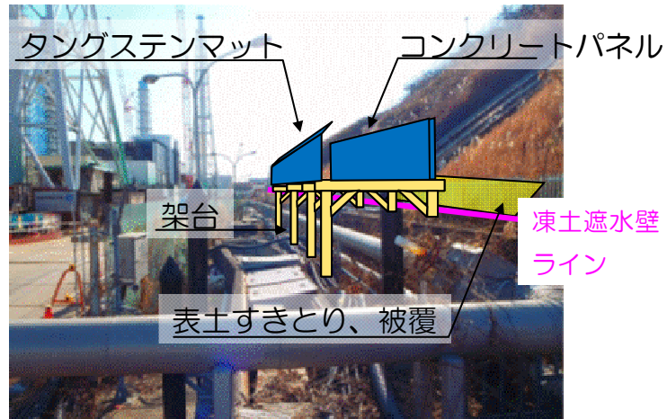
図 1 2 - 1 被ばく線量低減対策実施例 1 (既認可)
