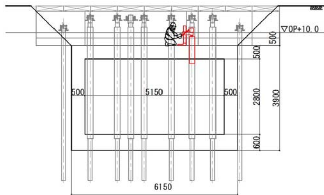
試削孔による溜まり水の確認方法
