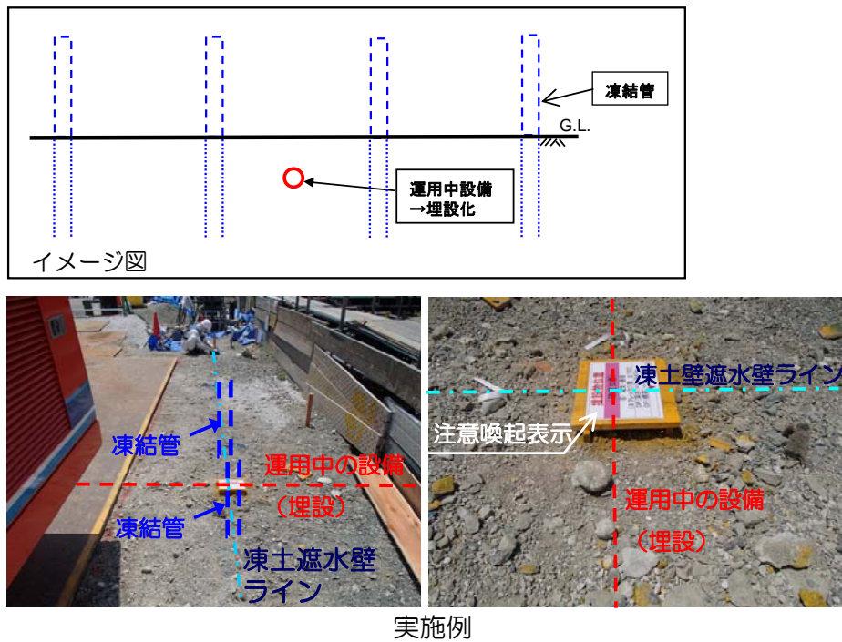
図 9-2 運用中の設備の防護パターン B (既認可)
