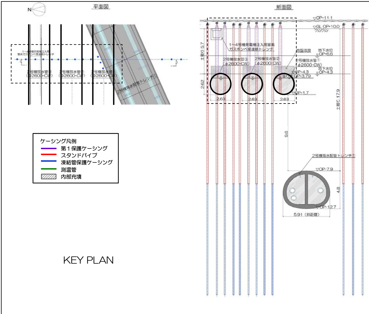
図7-17 【11-13】2号機放水管①②③ 施工方法（貫通施工）
