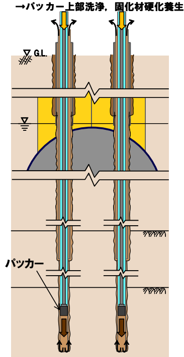
図3 頂版マルチステップ・底版内部充填工法の施工手順 (3)
