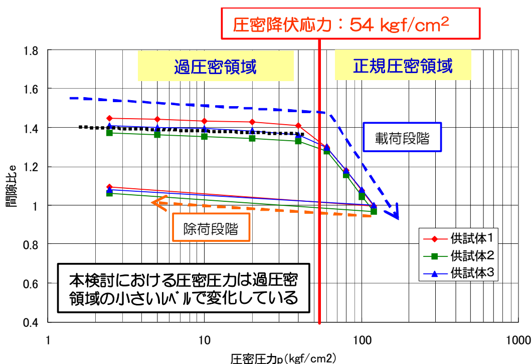
図2 圧密試験結果
