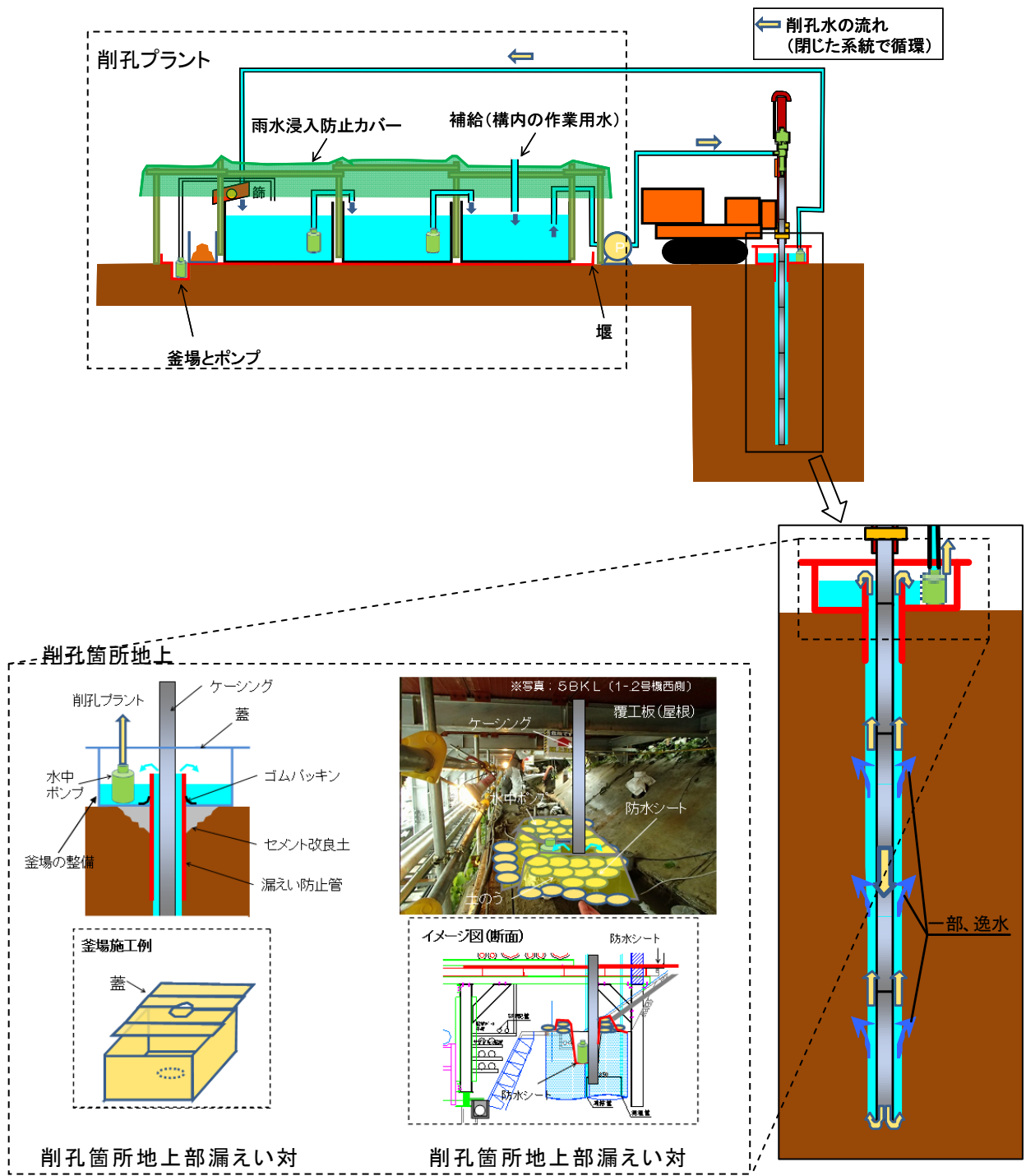
図 1 1 - 1 削孔水の漏えい対策イメージ (既認可)
