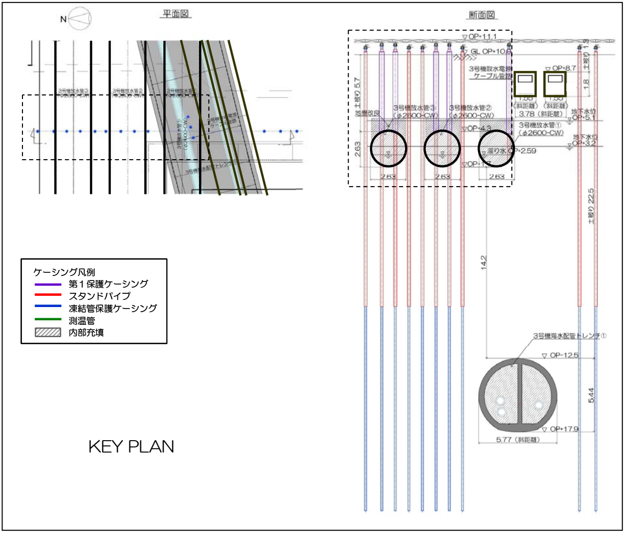
図7-12 【11-8】3号機放水管①②③ 施工方法（貫通施工）
