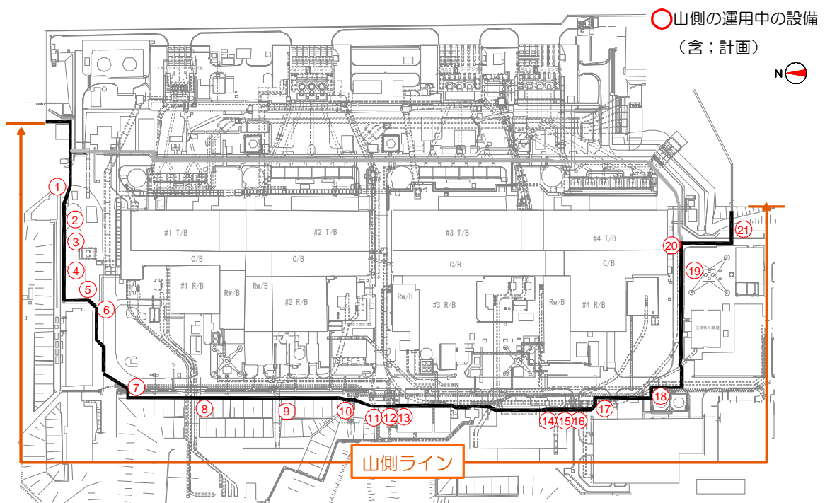
図 7 - 1 主な運用中の設備と凍土遮水壁の横断箇所（既認可）
