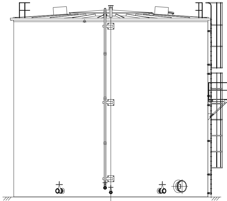
溶接型タンク概略図 (H1)
