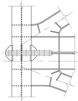
A-A 断面図
