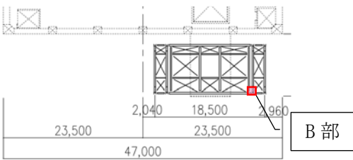
キープラン (O.P. 26.900 伏図)
