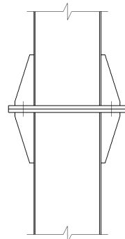
A-A 断面図
